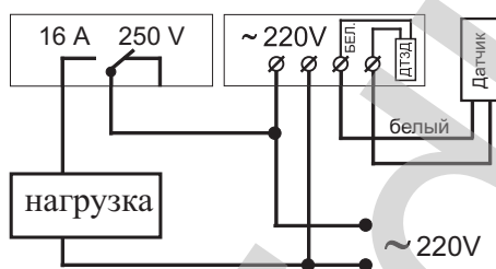
Рис.4 Схема подключения.
