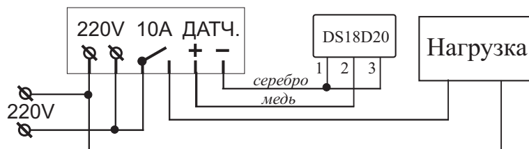
Рис.1. Схема подключения.
