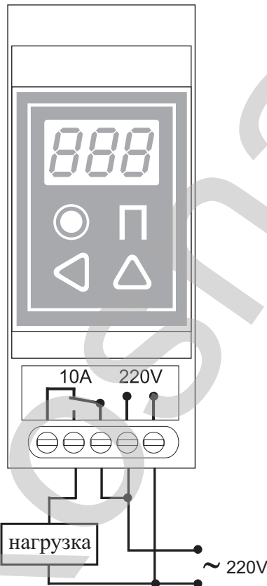
Рис.1 Схема подключения.
