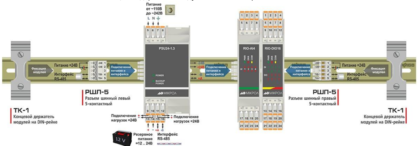
Рисунок 4.2 – Схема соединения блока питания с модулями УСО
