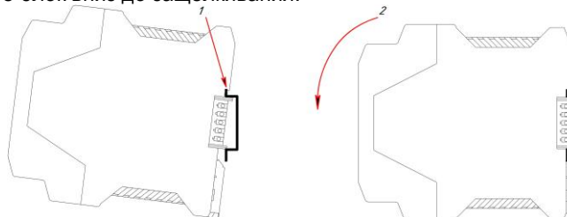
Рисунок 4.1 – Схема крепления блока питания на DIN-рельс
