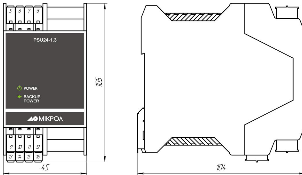
Рисунок 1.1 – Внешний вид и габаритные размеры PSU24-1.3
