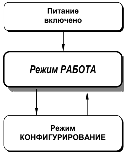
Рисунок 4.1 - Диаграмма уровней работы, защиты и настроек счетчика МТЛ-32Н
