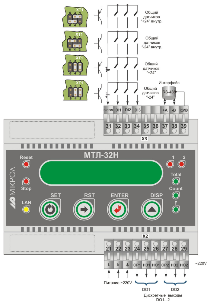
Рисунок Б.1.1 - Подключение внешних цепей счетчика МТЛ-32Н. Исполнение на напряжение 220 В переменного тока
