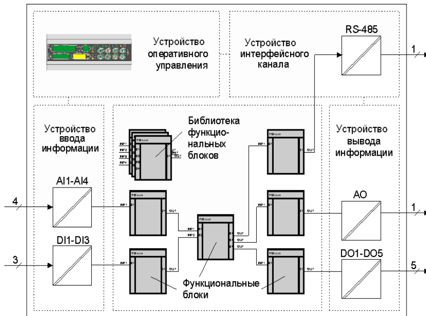
Рисунок 4.1 - Архитектура контроллера МИК-52Н
