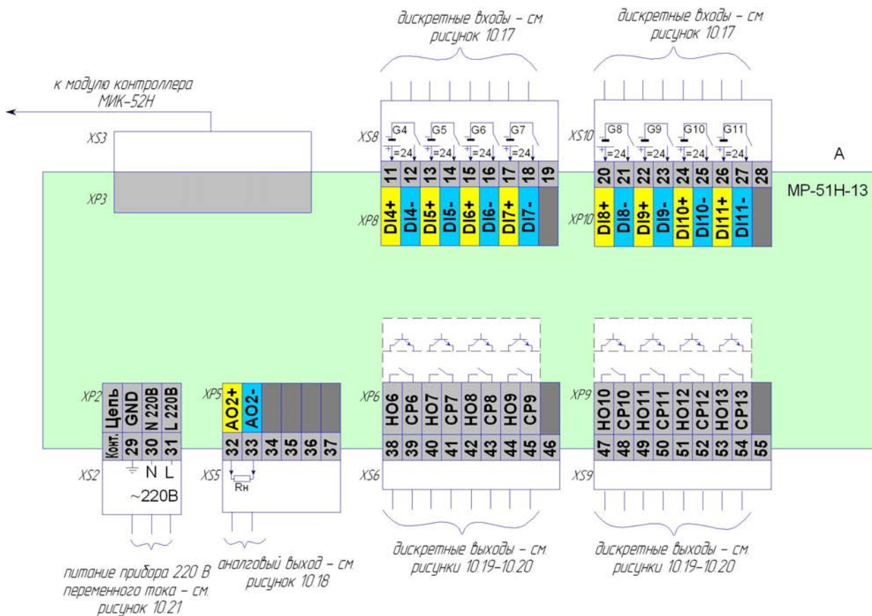
Рисунок 10.12.1 - Схема подключения сигналов модуля расширения MP-51H-13 с питанием 220В переменного тока, внешний вид
