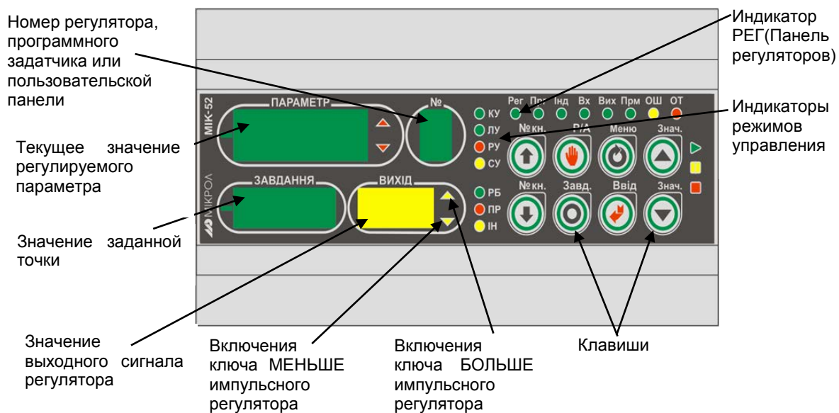
Рисунок 6.4 - Лицевая панель в режиме оперативного управления контурами регулирования
