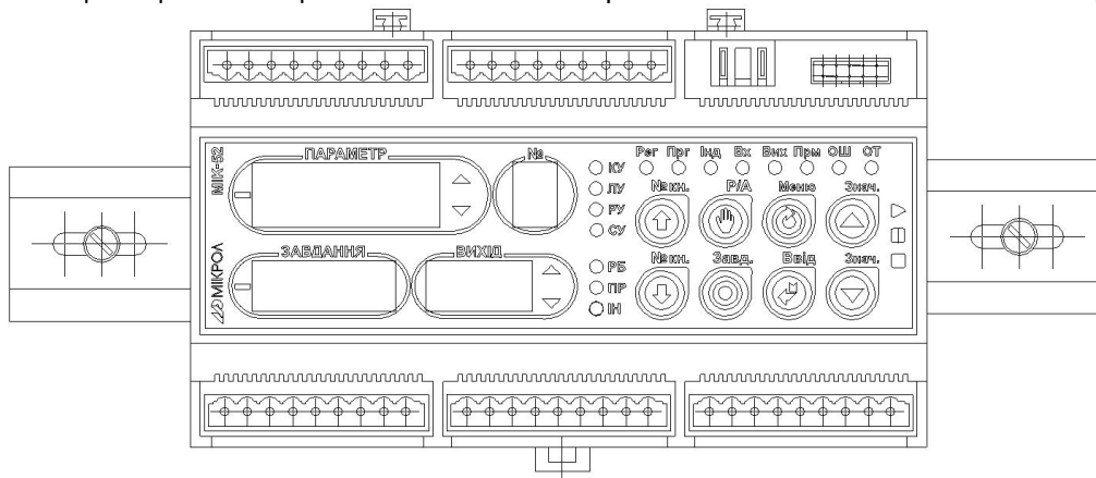
Рисунок 9.1 – Положение МИК-52Н при монтаже на DIN-Рельс
