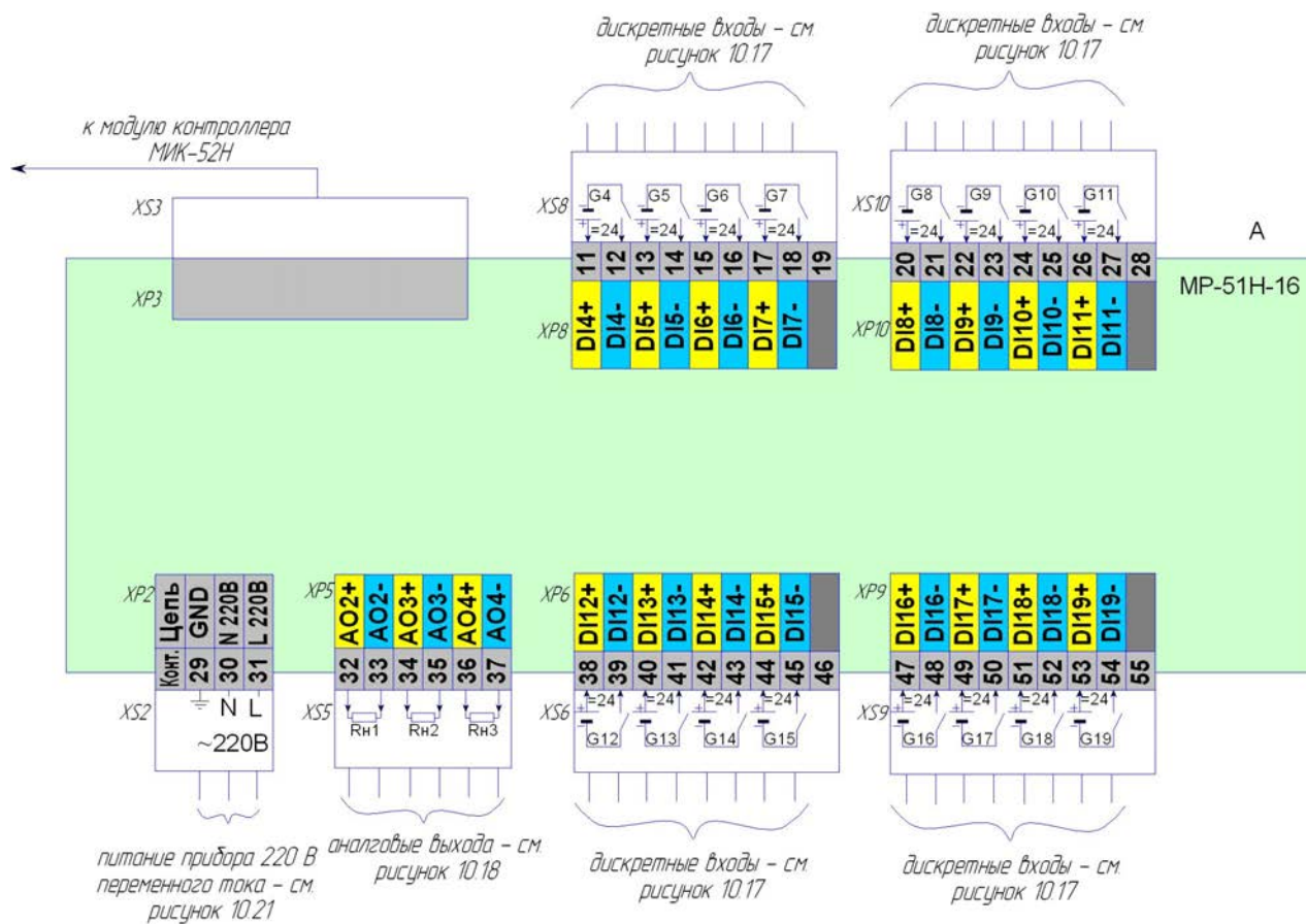
Рисунок 10.14.1 - Схема подключения сигналов модуля расширения МР-51Н-16 с питанием 220В переменного тока, внешний вид
