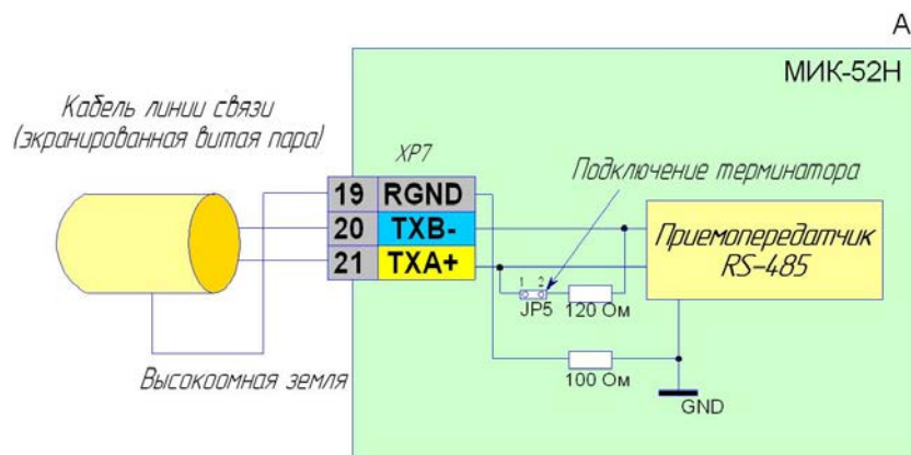
Рисунок 10.10 – Схема подключения интерфейса
