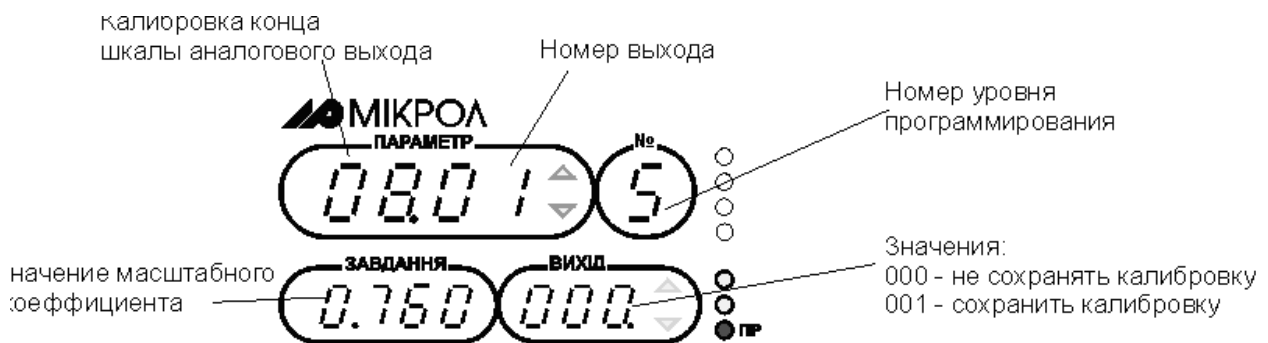
Рис 11.2 Внешний вид индикаторов при калибровке конечного значения аналогового выхода
