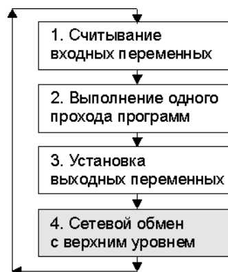
Рисунок 4.8 - Циклограмма работы контроллера
