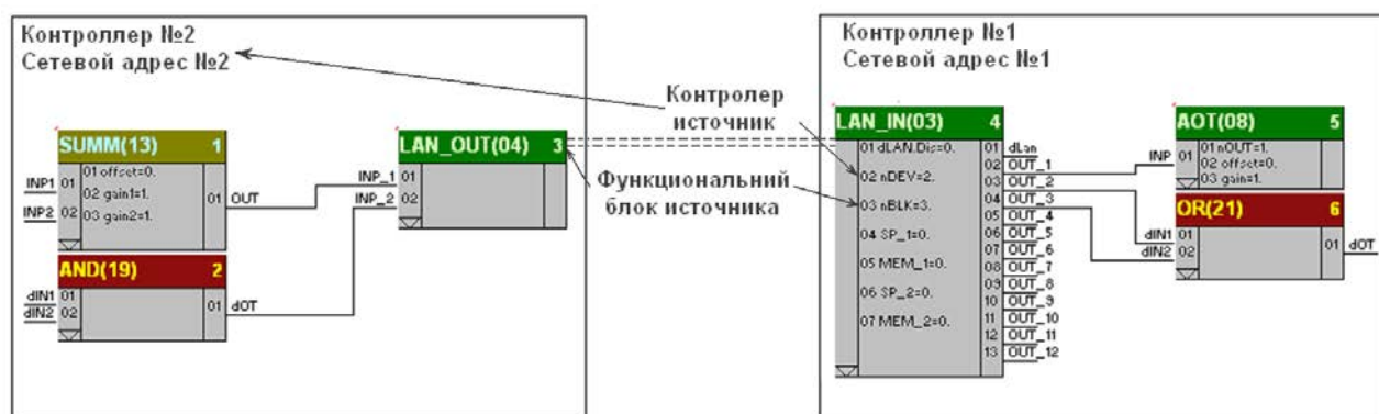
Рисунок 5.2 - Связь двух контроллеров через функциональные блоки интерфейсного ввода-вывода
