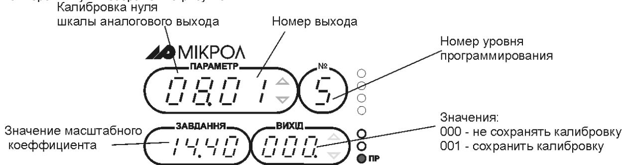
Рис 11.1 Внешний вид индикаторов при калибровке нуля аналогового выхода
