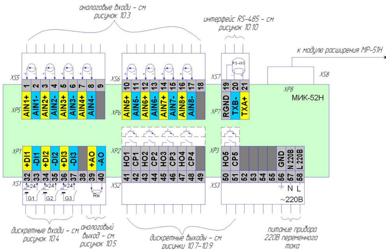
Рисунок 10.1 - Контроллер малоканальный микропроцессорный многофункциональный МИК-52Н с питанием 220 В переменного тока, внешний вид схем подключения
