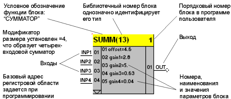
Рисунок 4.2 - Функциональный блок сумматора
