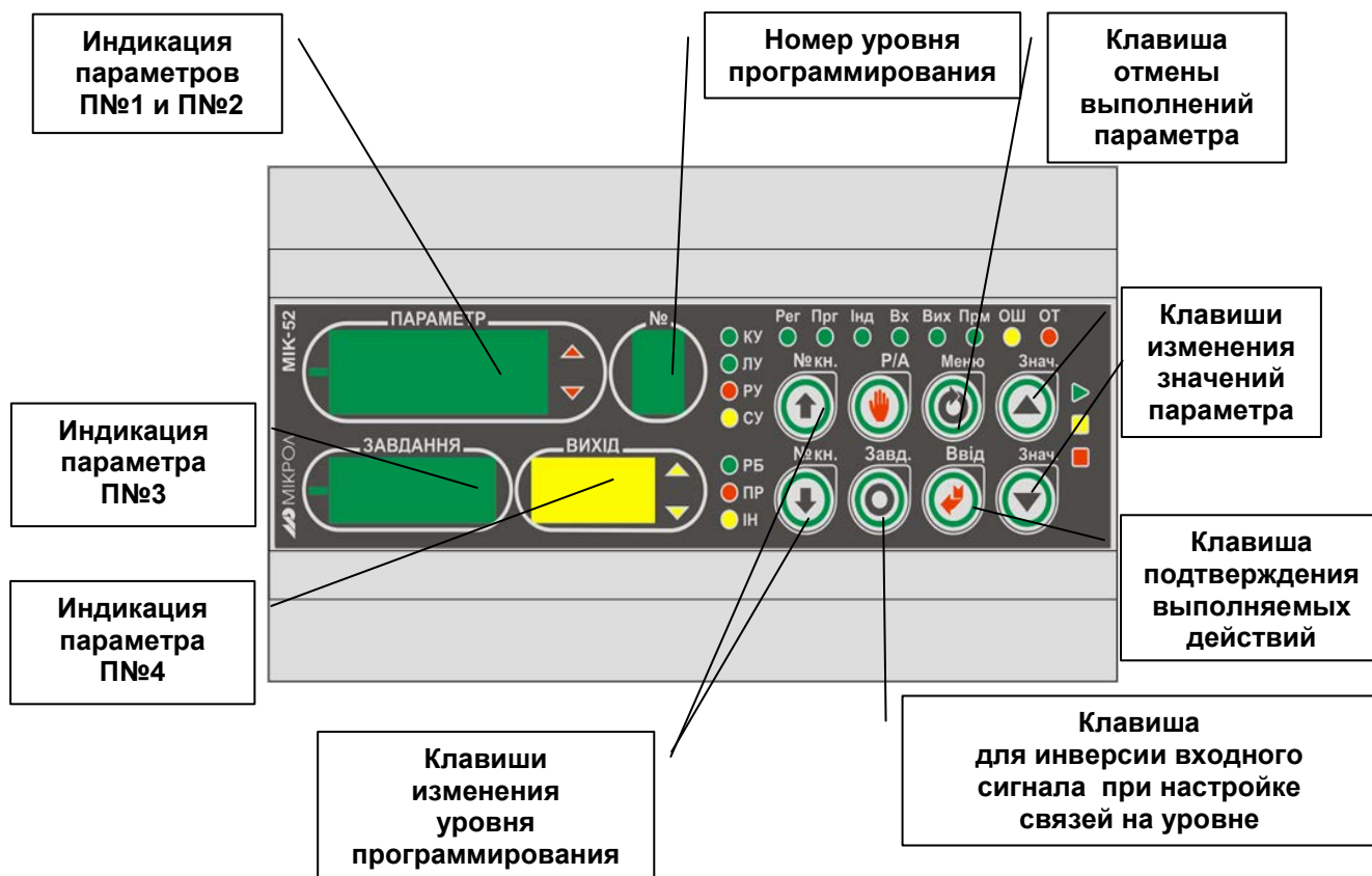
Рисунок 7.1 - Лицевая панель контроллера МИК-52Н в режиме программирования
