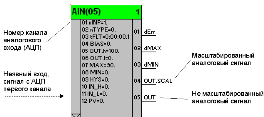
Рисунок 4.3 - Функциональный блок аналогового ввода с неявными входами
