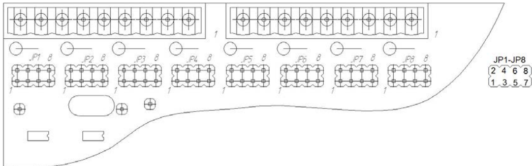
Рисунок 10.3.1 – Положение перемычек аналоговых входов
