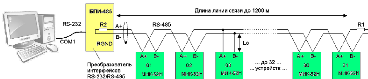
Рисунок 5.1 - Структурная схема подключения интерфейсных цепей
