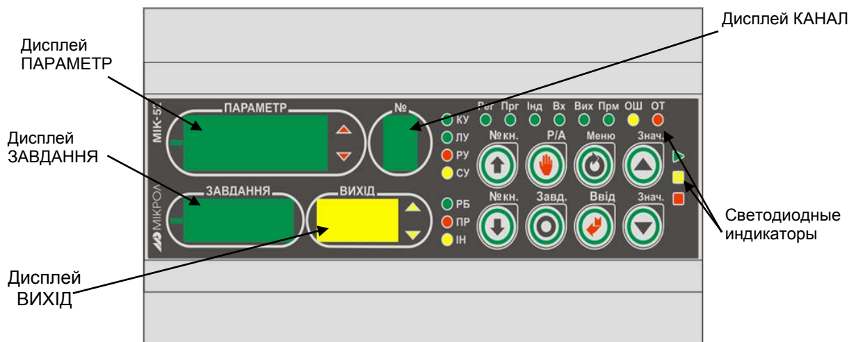
Рисунок 6.1 - Элементы оперативного управления
