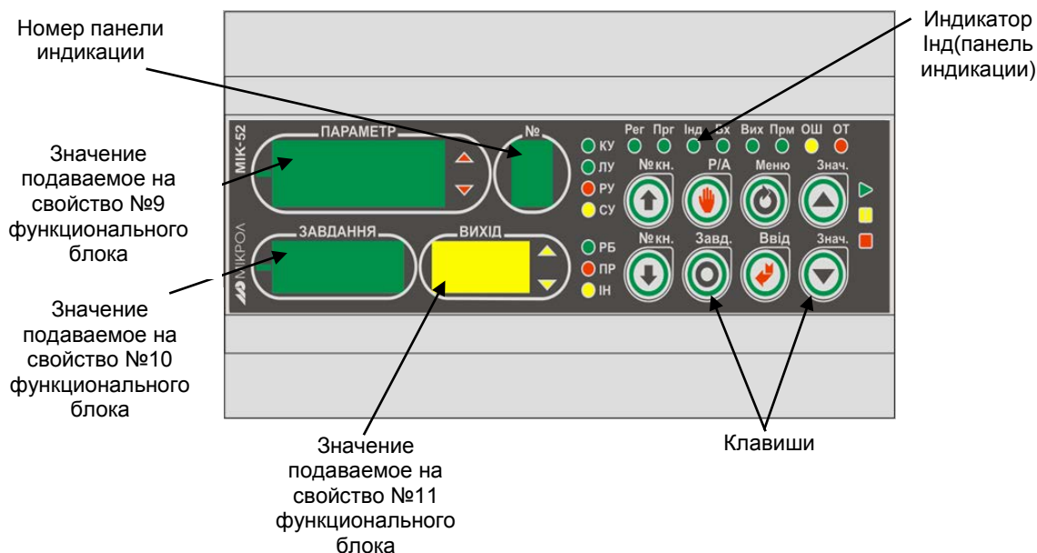
Рисунок 6.8 - Лицевая панель в режиме оперативного управления программным задатчиком
