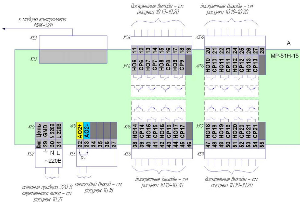
Рисунок 10.13.1 - Схема подключение сигналов модуля расширения МР-51Н-15 с питанием 220В переменного тока, внешний вид
