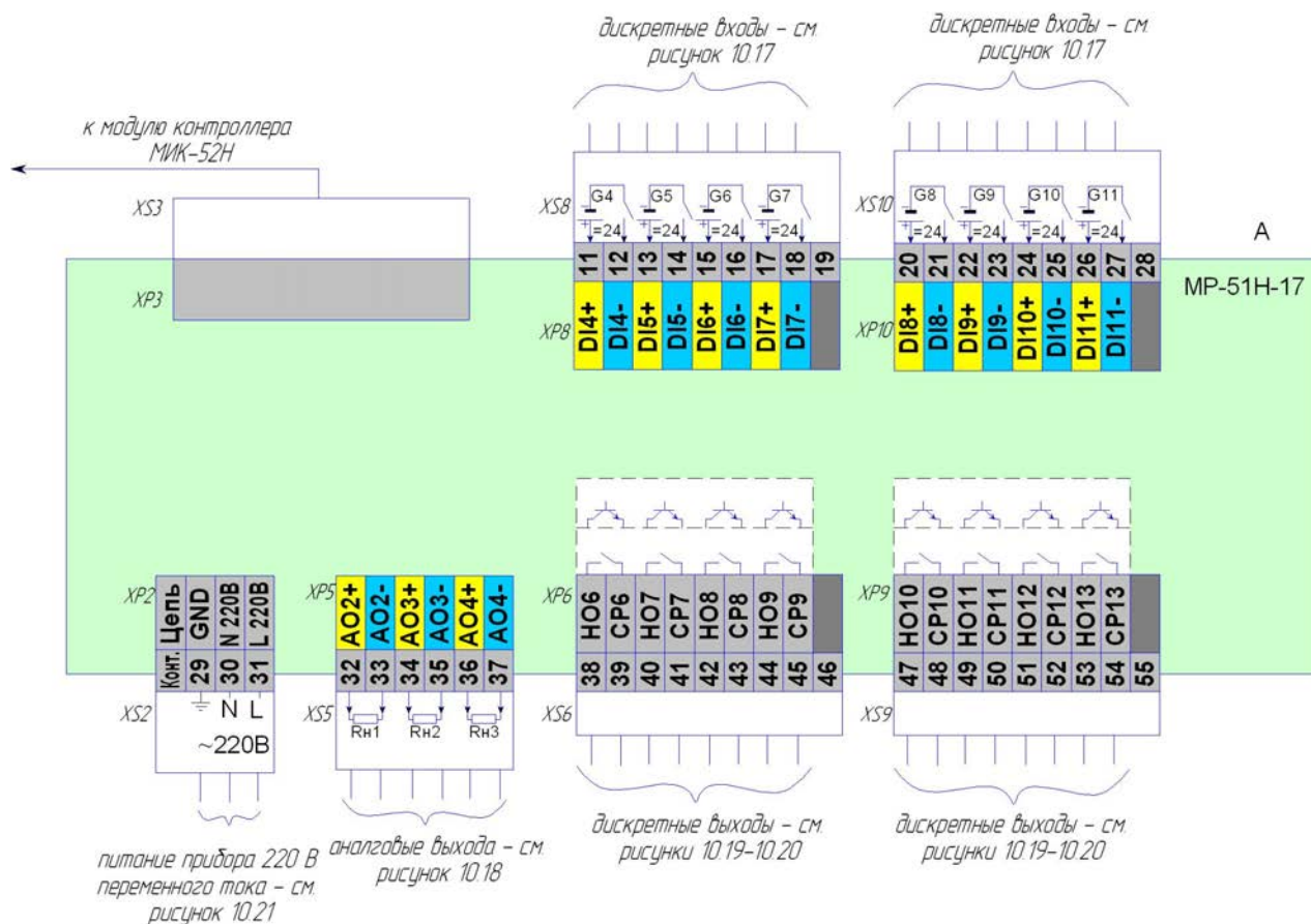
Рисунок 10.15.1 - Схема подключения сигналов модуля расширения МР-51Н-17 с питанием 220В переменного тока, внешний вид
