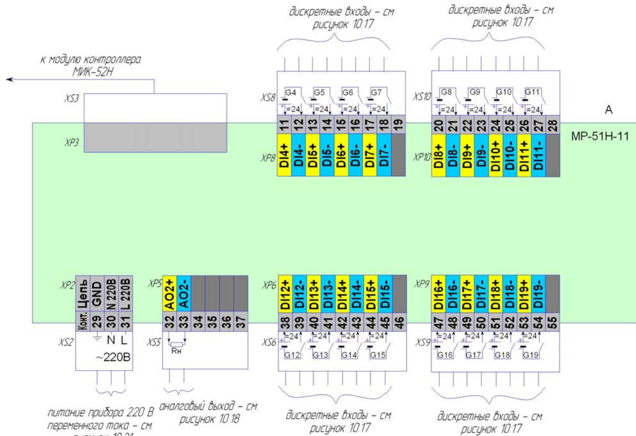
Рисунок 10.11.1 - Схема подключения сигналов модуля расширения МР-51Н-11 с питанием 220В переменного тока, внешний вид
