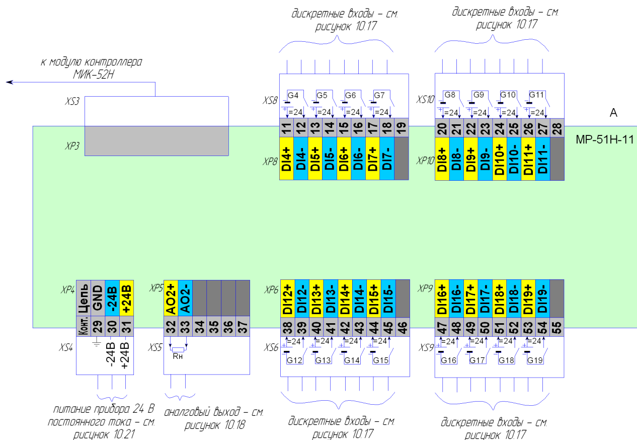
Рисунок 10.11.2 - Схема подключения сигналов модуля расширения MP-51H-11 с питанием 24В постоянного тока, внешний вид
