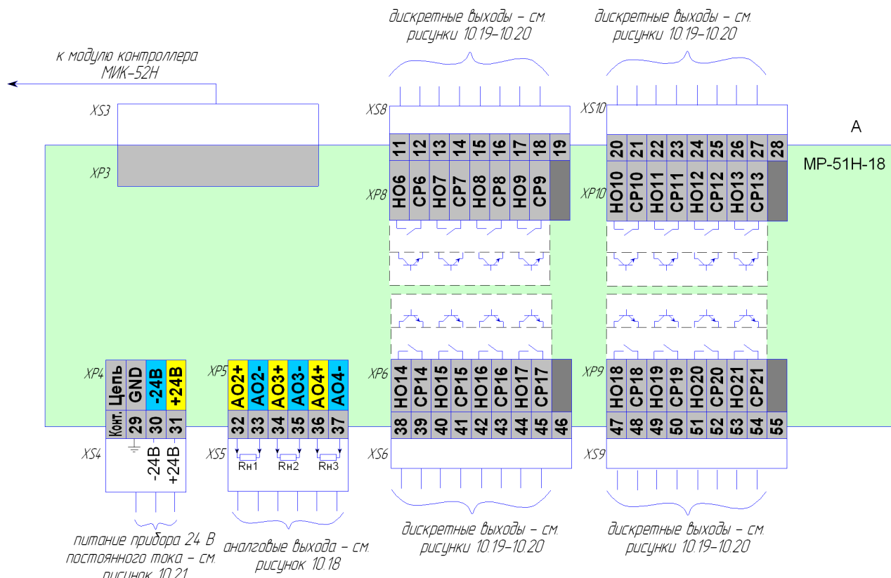
Рисунок 10.16.2 - Схема подключения сигналов модуля расширения MP-51H-18 с питанием 24В постоянного тока, внешний вид
