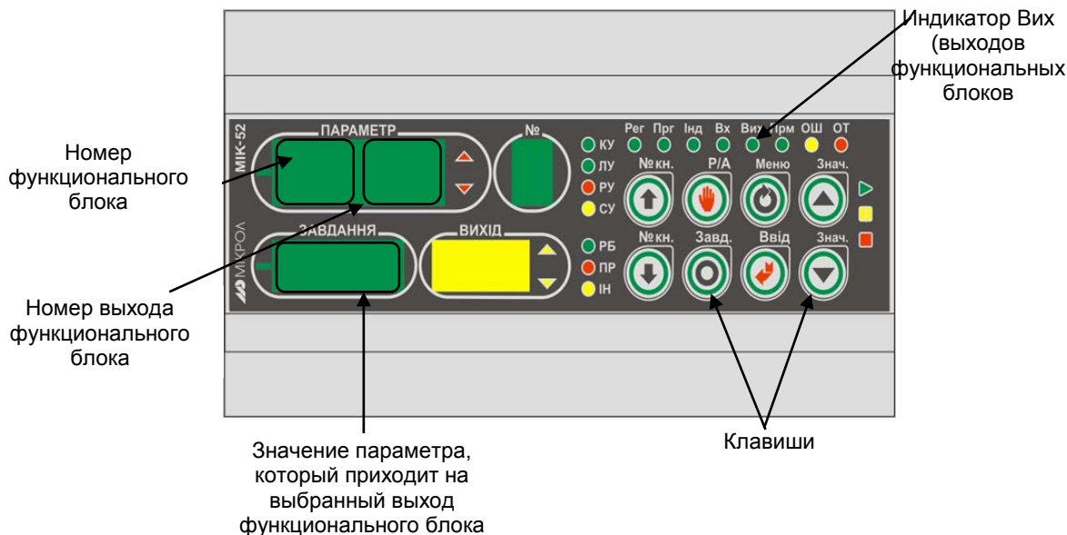
Рисунок 6.10 - Лицевая панель в режиме индикации выходных параметров функциональных блоков
