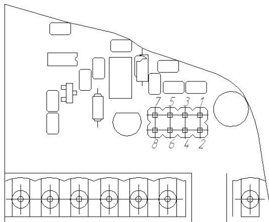
Рисунок 10.6– Положение перемычек для настройки аналогового выхода
