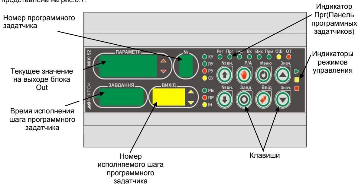
Рисунок 6.7 - Лицевая панель в режиме оперативного управления программным задатчиком
