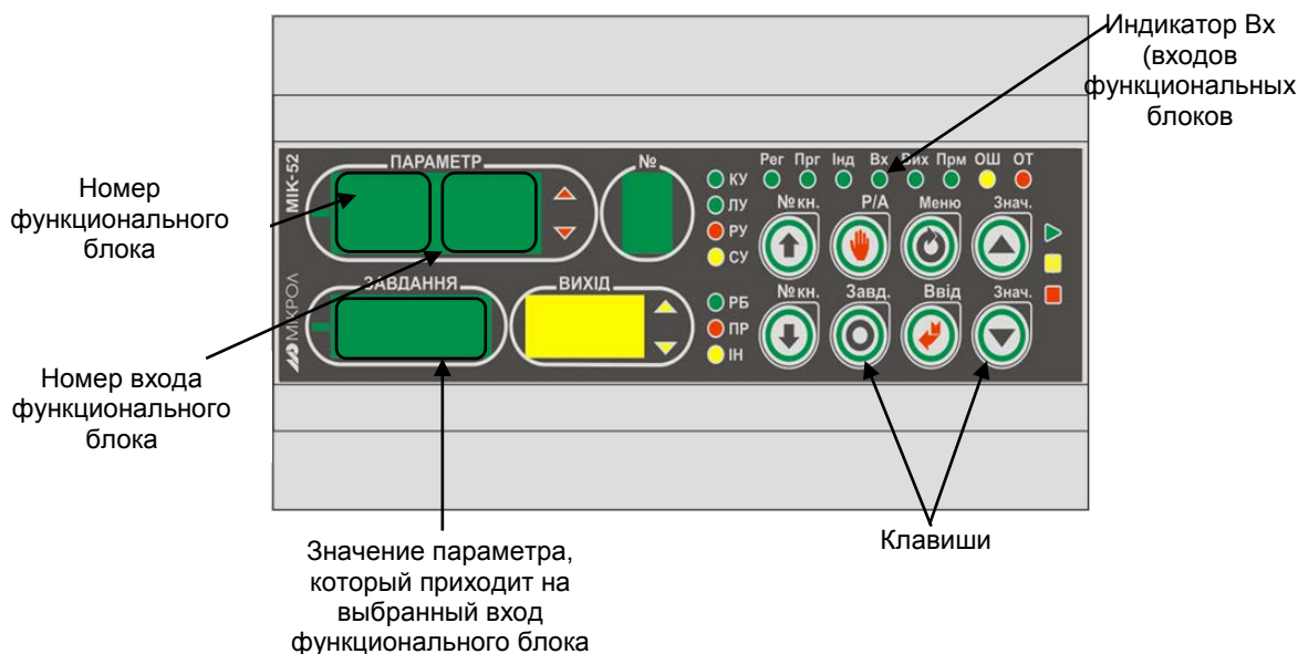
Рисунок 6.9 - Лицевая панель в режиме индикации входных параметров функциональных блоков
