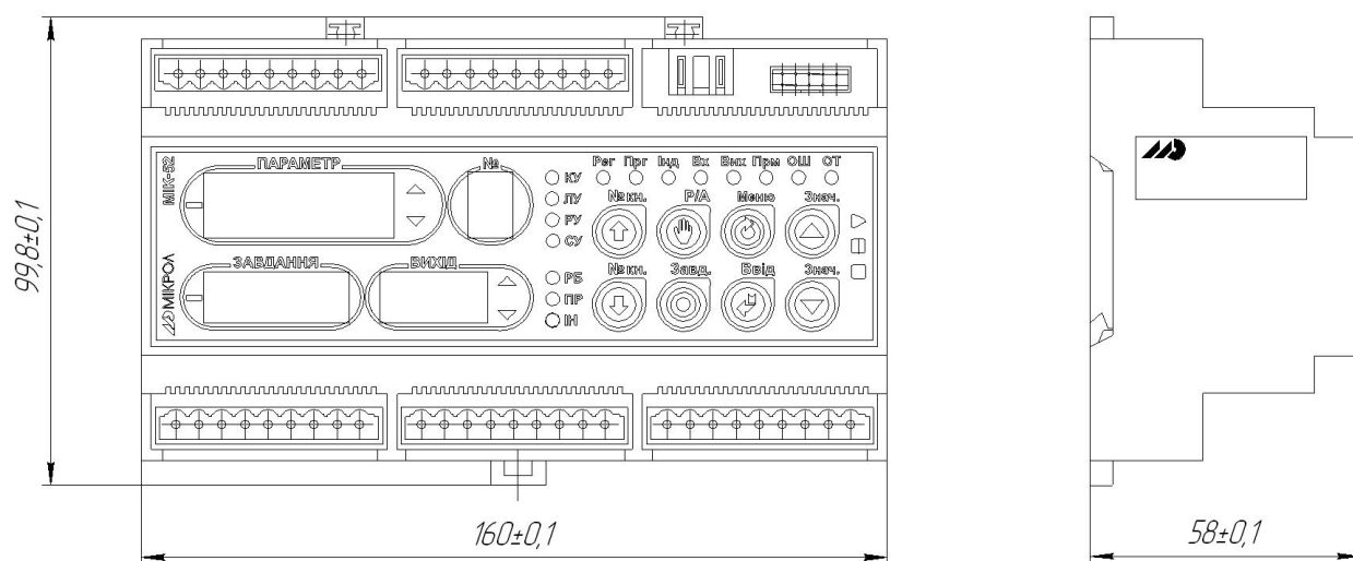
Рисунок 9.2- Контроллер малоканальный микропроцессорный многофункциональный МИК-52Н, внешний вид и габаритные размеры
