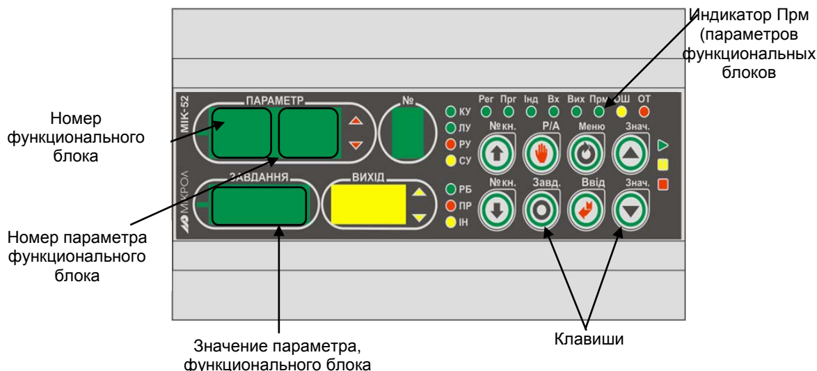
Рисунок 6.11 - Лицевая панель в режиме индикации параметров функциональных блоков
