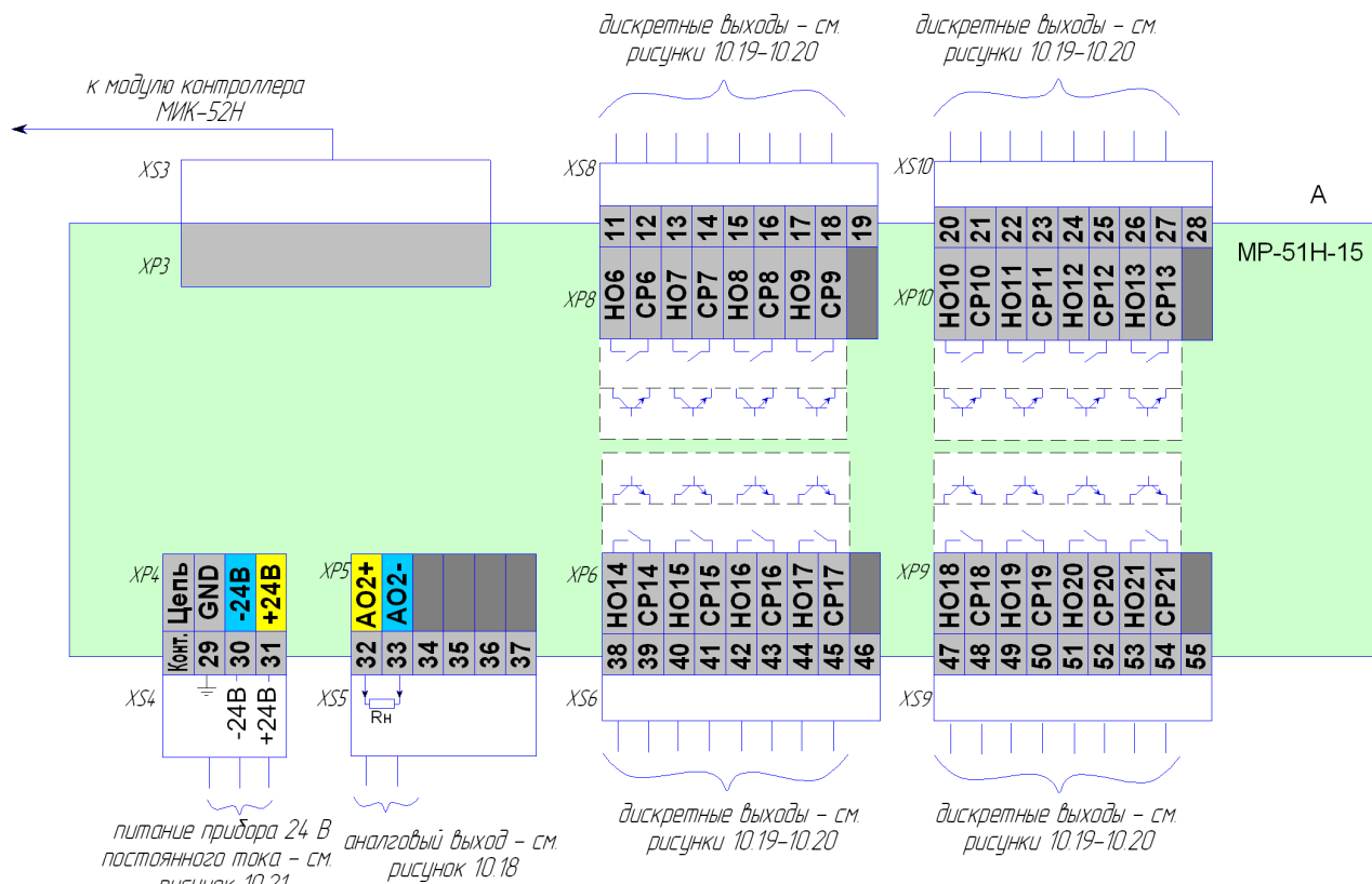
Рисунок 10.13.2 - Схема подключения сигналов модуля расширения MP-51H-15 с питанием 24В постоянного тока, внешний вид
