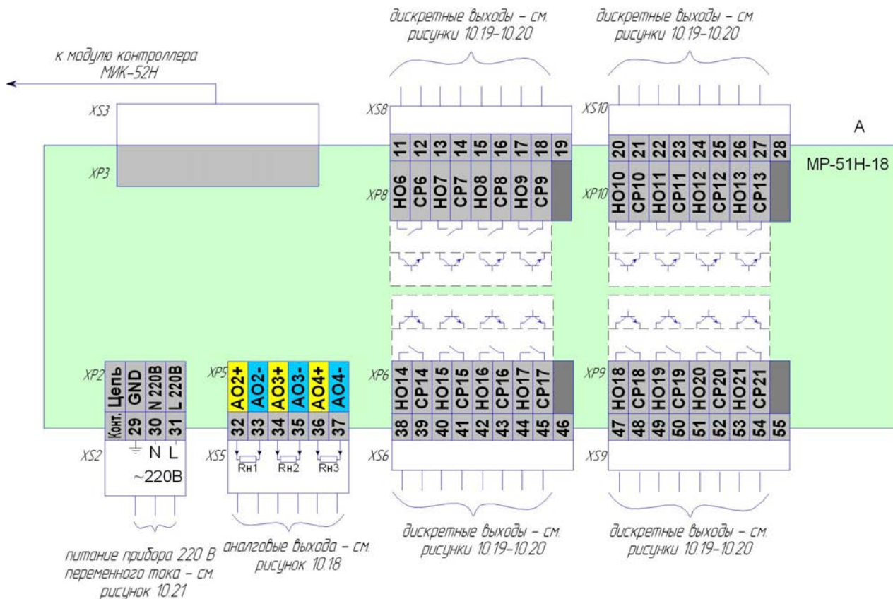
Рисунок 10.16.1 - Схема подключения сигналов модуля расширения МР-51Н-18 с питанием 220В переменного тока, внешний вид
