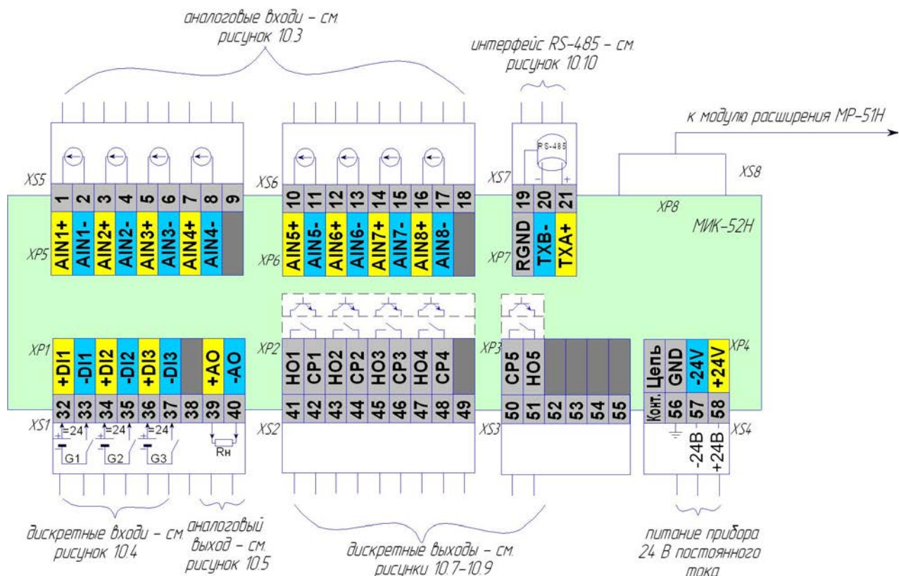
Рисунок 10.2 - Контроллер малоканальный микропроцессорный многофункциональный МИК-52Н с питанием 24 В постоянного тока, внешний вид схем подключения
