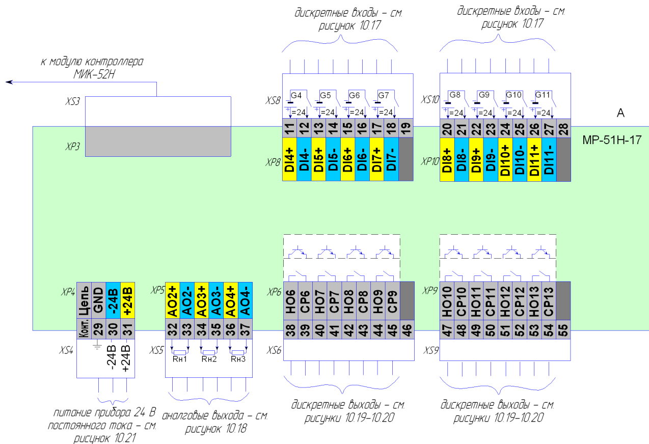
Рисунок 10.15.2 - Схема подключения сигналов модуля расширения MP-51H-17 с питанием 24В постоянного тока, внешний вид
