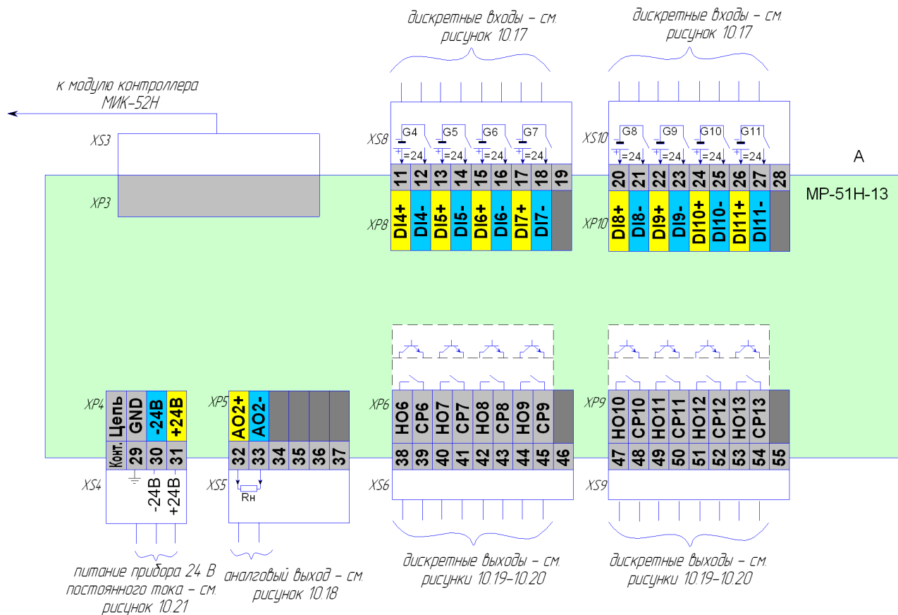
Рисунок 10.12.2 - Схема подключения сигналов модуля расширения MP-51H-13 с питанием 24В постоянного тока, внешний вид
