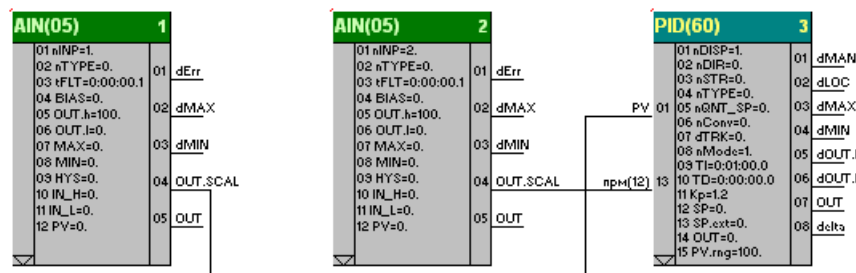
Рисунок 4.6 – Связные параметры
