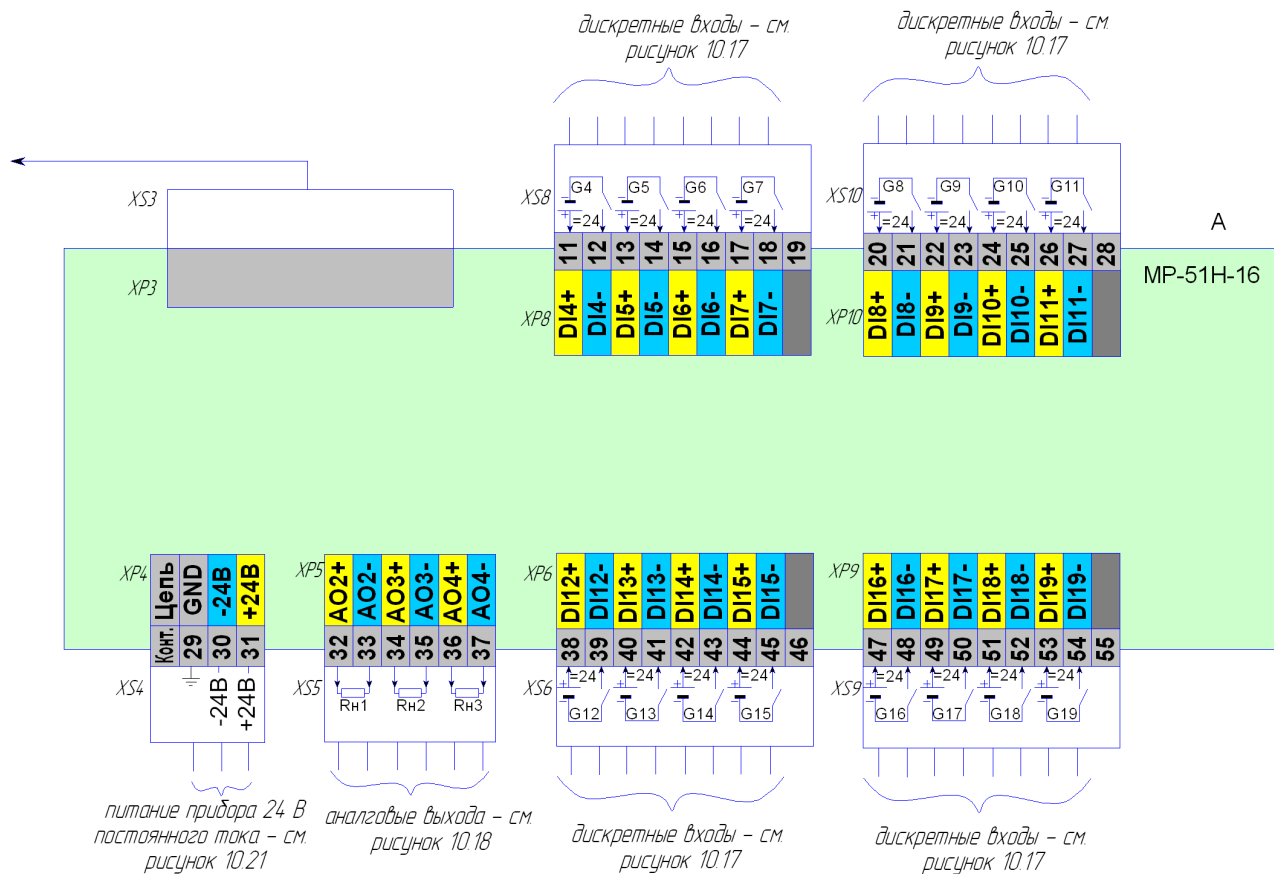
Рисунок 10.14.2 - Схема подключения сигналов модуля расширения MP-51H-16 с питанием 24В постоянного тока, внешний вид
