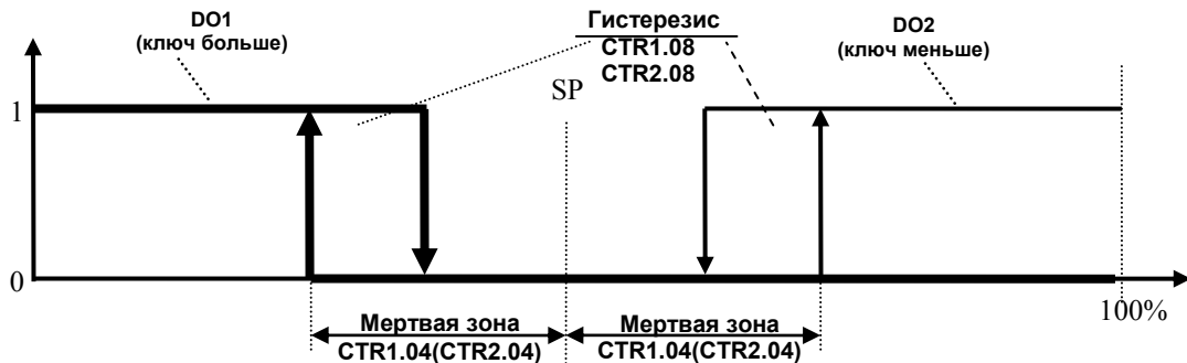
Рисунок 3.6 - График работы дискретных выходов 3-х позиционного регулятора с использованием зоны нечувствительности CTR1.04(CTR2.04)
