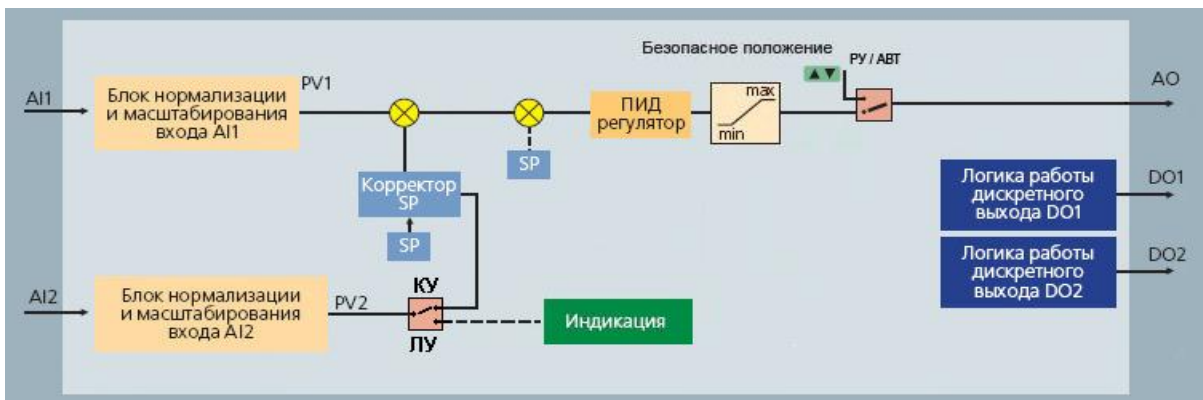
Рисунок 3.8 – Структурная схема регулятора с внешней коррекцией задания
