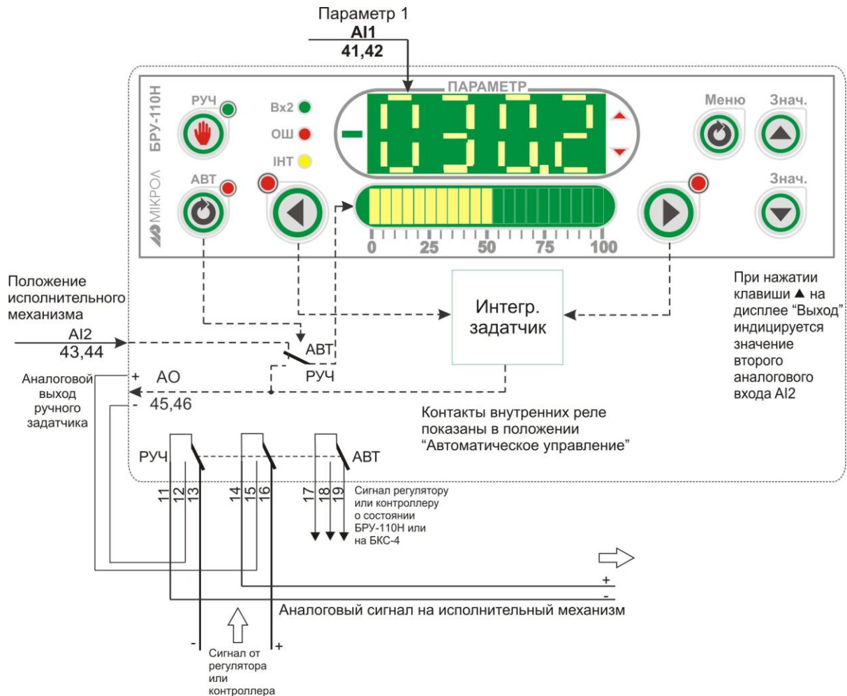
Рисунок 4.8 - Блок-схема режима 1
