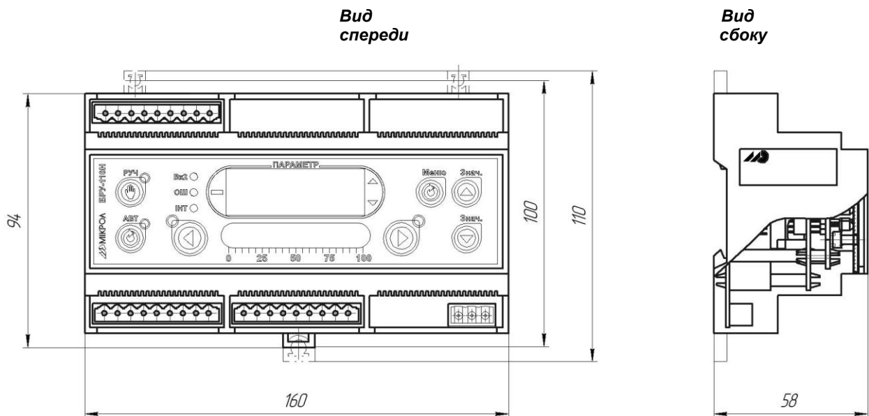
Рисунок А.2 - Габаритные размеры
