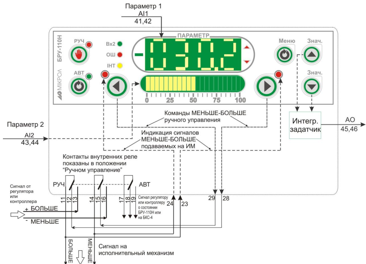
Рисунок 4.17 - Блок-схема режима 7
