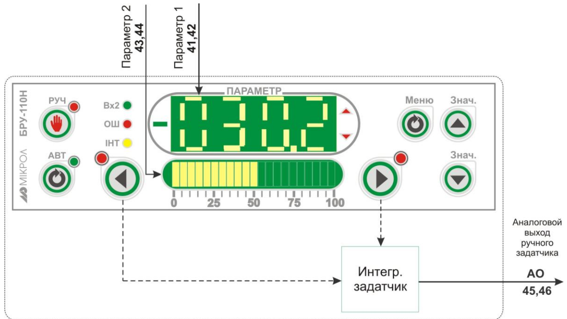
Рисунок 4.7 - Блок-схема режима 0
