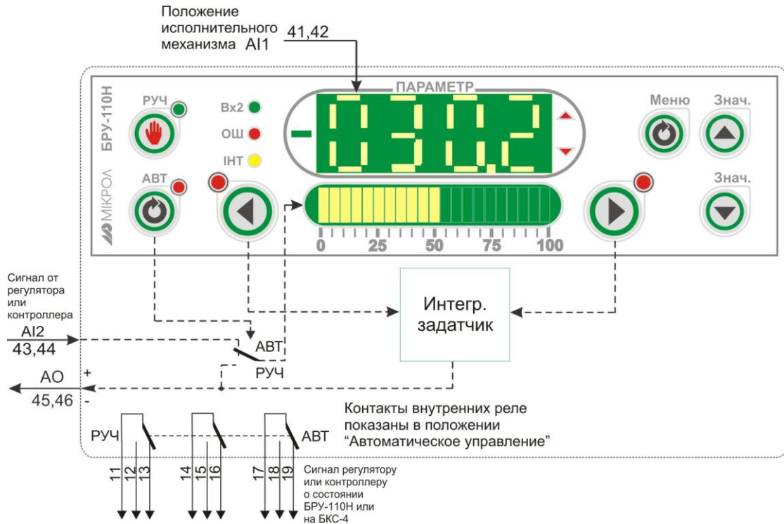
Рисунок 4.23 - Блок-схема режима 11
