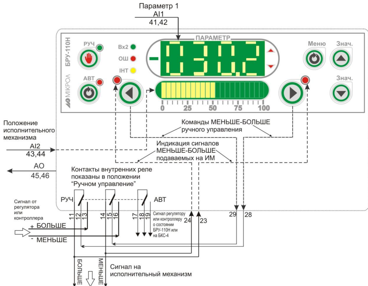
Рисунок 4.11 - Блок-схема режима 3
