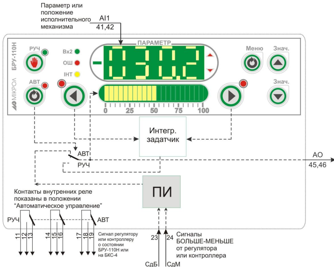
Рисунок 4.12 - Блок-схема режима 4
