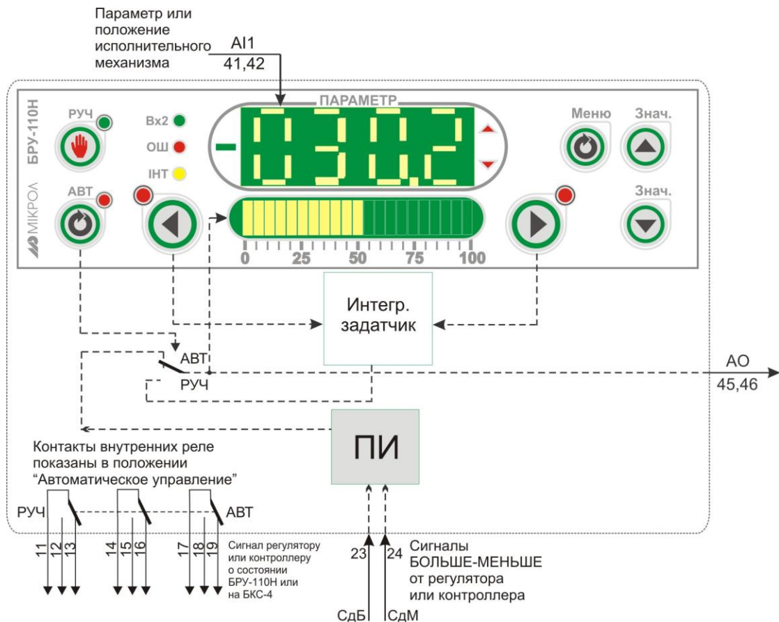
Рисунок 4.19 - Блок-схема режима 9
