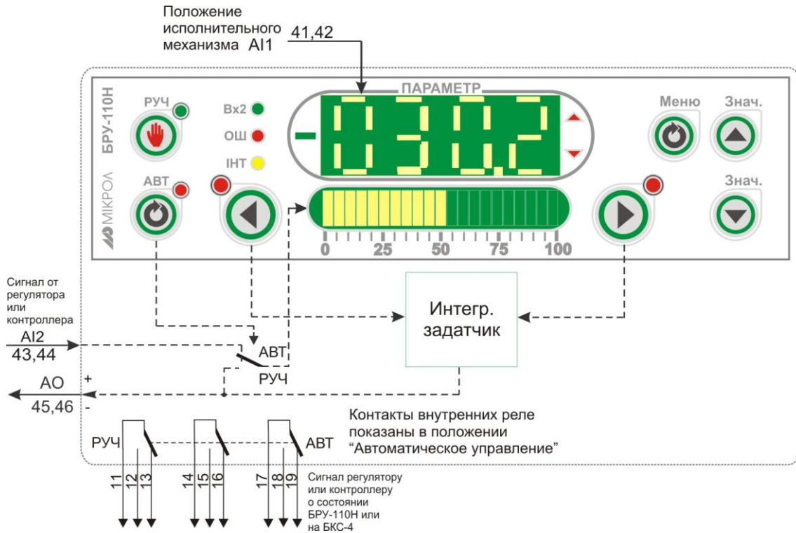
Рисунок 4.10 - Блок-схема режима 2
