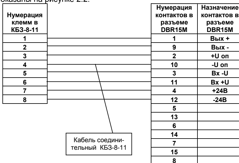
Рисунок 2.2 - Схема распайки кабеля клеммно-блочного соединителя КБЗ-8-11 и внешние сигналы БПТ-2
