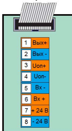
Рисунок 4.3 Схема электрических подключений к КБЗ-16-11
