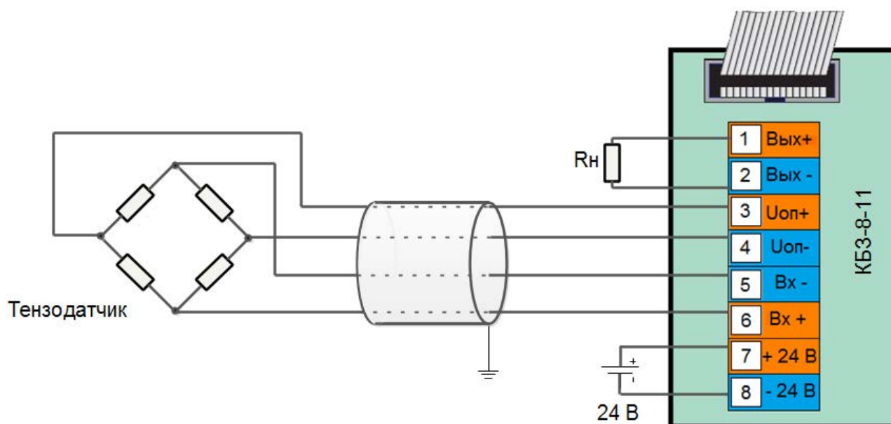
Рисунок 2.1 - Схема внешних соединений БПТ-2 с использованием КБЗ-8-11
