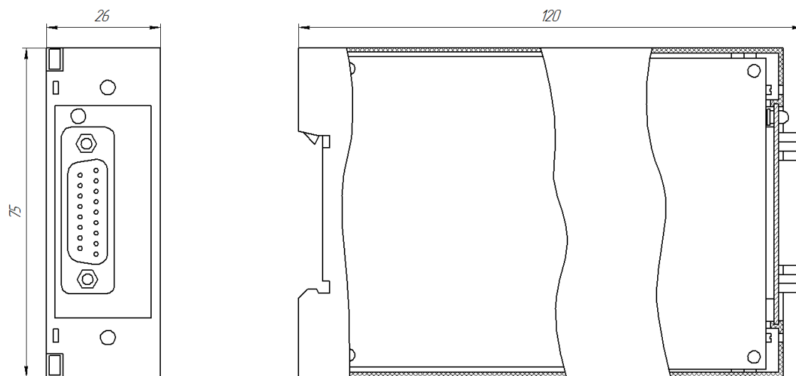
Рисунок 1.1 - Внешний вид и габаритные размеры БПТ-2
