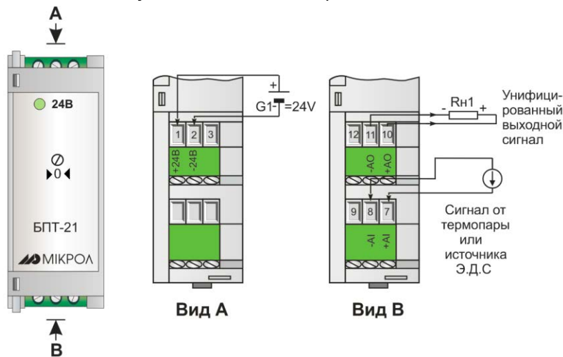
Рисунок 4.4 Схема электрических подключений.
