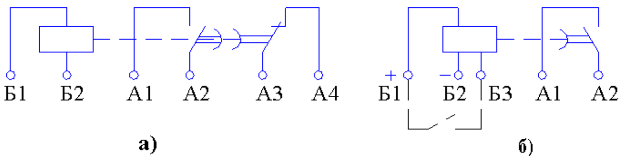
Рисунок 2 – Функциональные диаграммы реле
