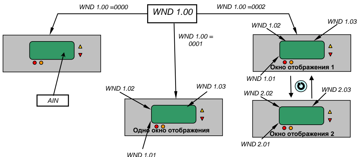
Рисунок 5.7 – Блок-схема выбора вариантов отображения измерительного параметра
