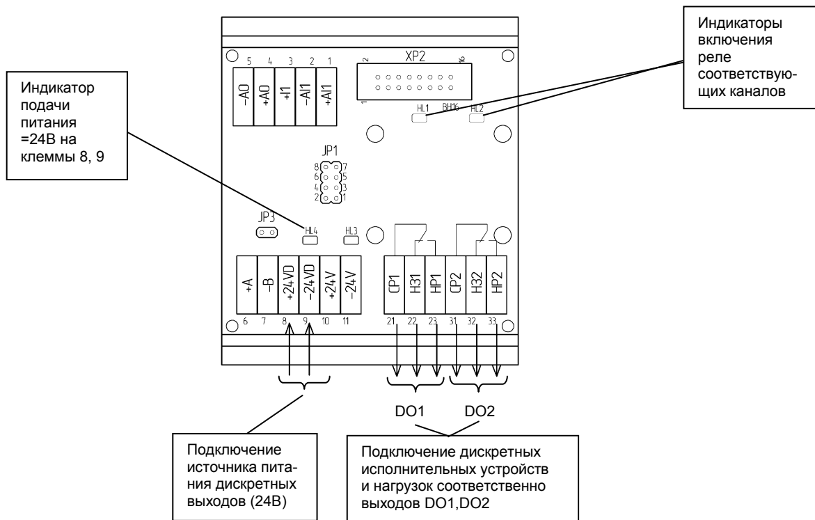
Рисунок Б.15 - Подключение дискретных нагрузок с помощью КБЗ-17P-01
