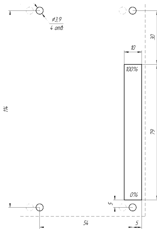
Рисунок А.4 - Рекомендуемый вырез в щите для вертикального положения индикатора ИТМ-1-01-31
