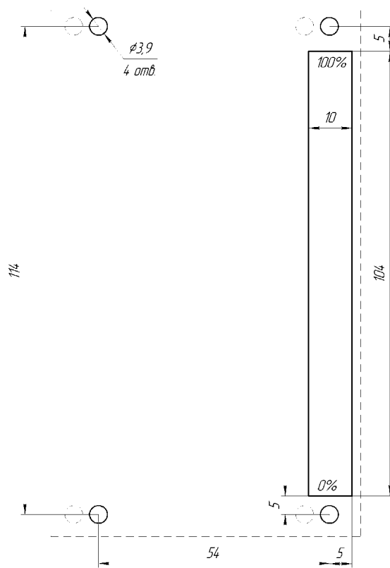
Рисунок А.8 - Рекомендуемый вырез в щите для вертикального положения индикатора ИТМ-1-01-41
