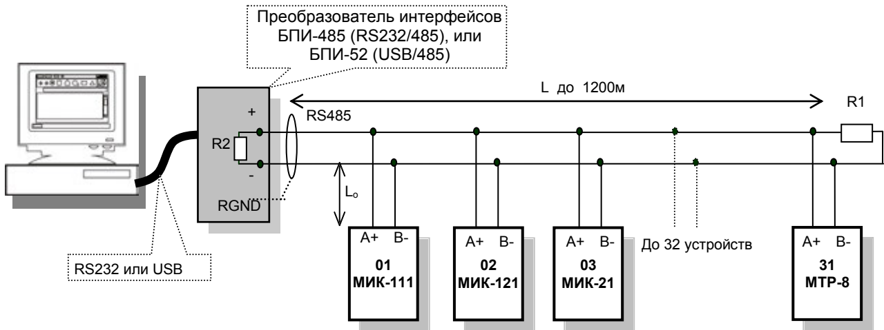
Рисунок Б.4 - Организация интерфейсной связи между компьютером и регуляторами
