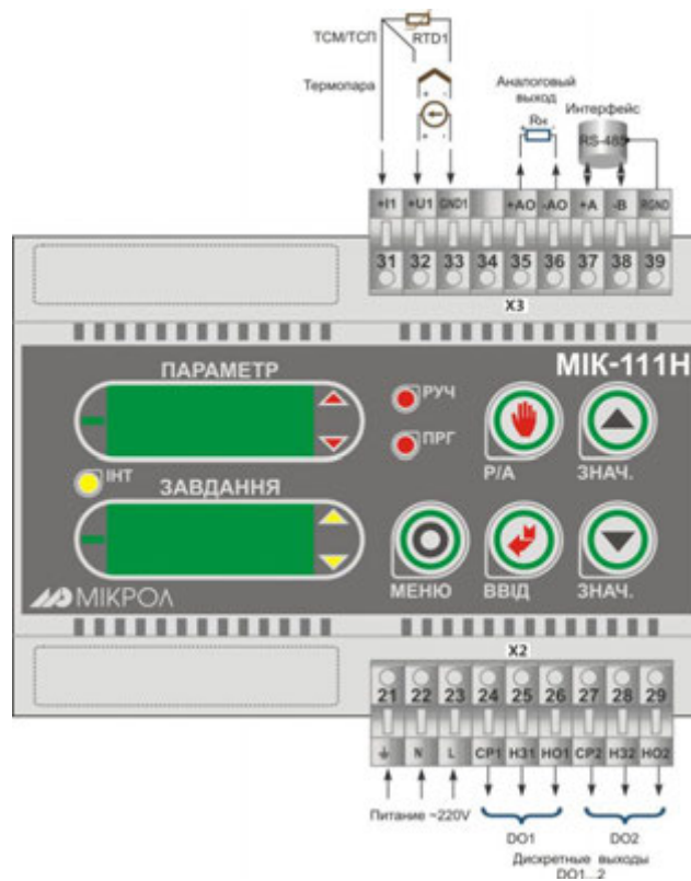
Рисунок Б.1 - Подключение внешних цепей к регулятору МИК-111Н
