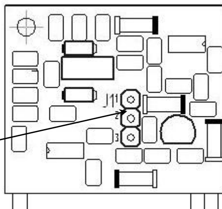
Рисунок 4.6 – Положение переключек на плате процессора а) основная плата процессора; б) плата аналогового выхода.
