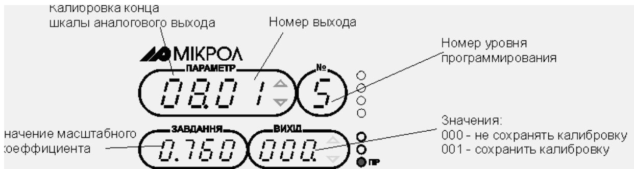
Рис 11.4.2.2 Внешний вид индикаторов при калибровке конечного значения аналогового выхода
