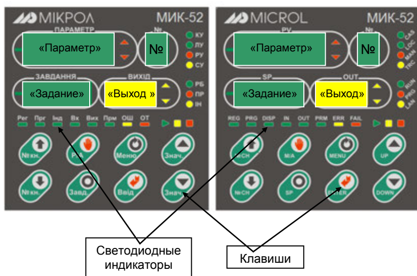
Рисунок 6.1 - Элементы оперативного управления
