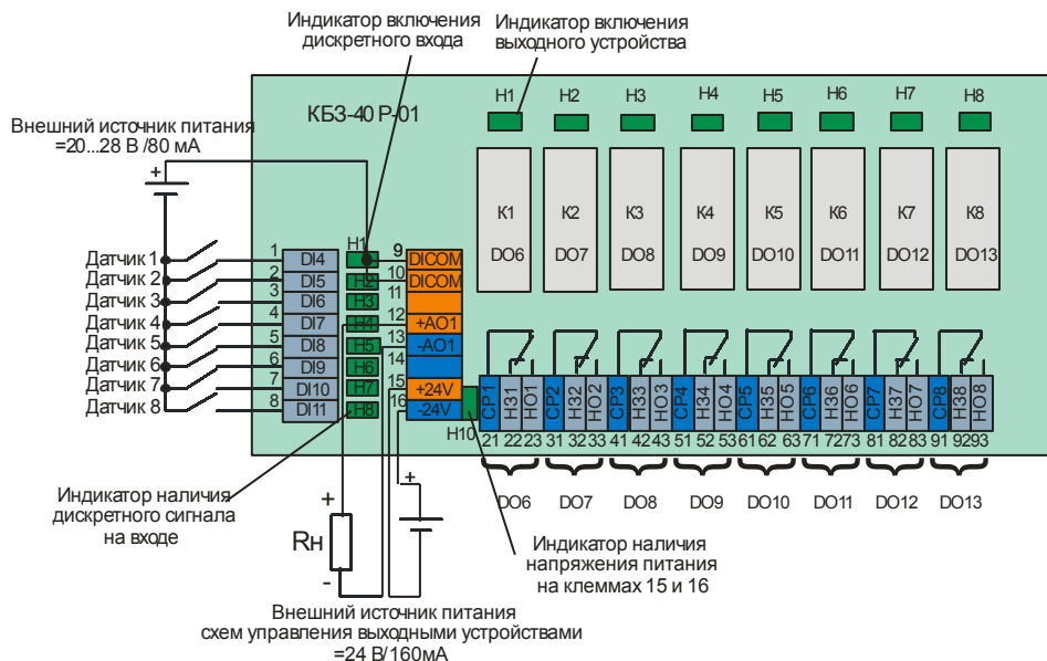
Рисунок 10.4.10 - Подключение сигналов модуля расширения МР-51-13 с помощью клеммно-блочного соединителя КБЗ-40Р-01
