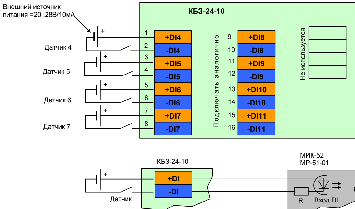
Рисунок 10.4.1.1 - Подключение сигналов модуля расширения МР-51-01 с помощью клеммно-блочного соединителя КБЗ-24-10
