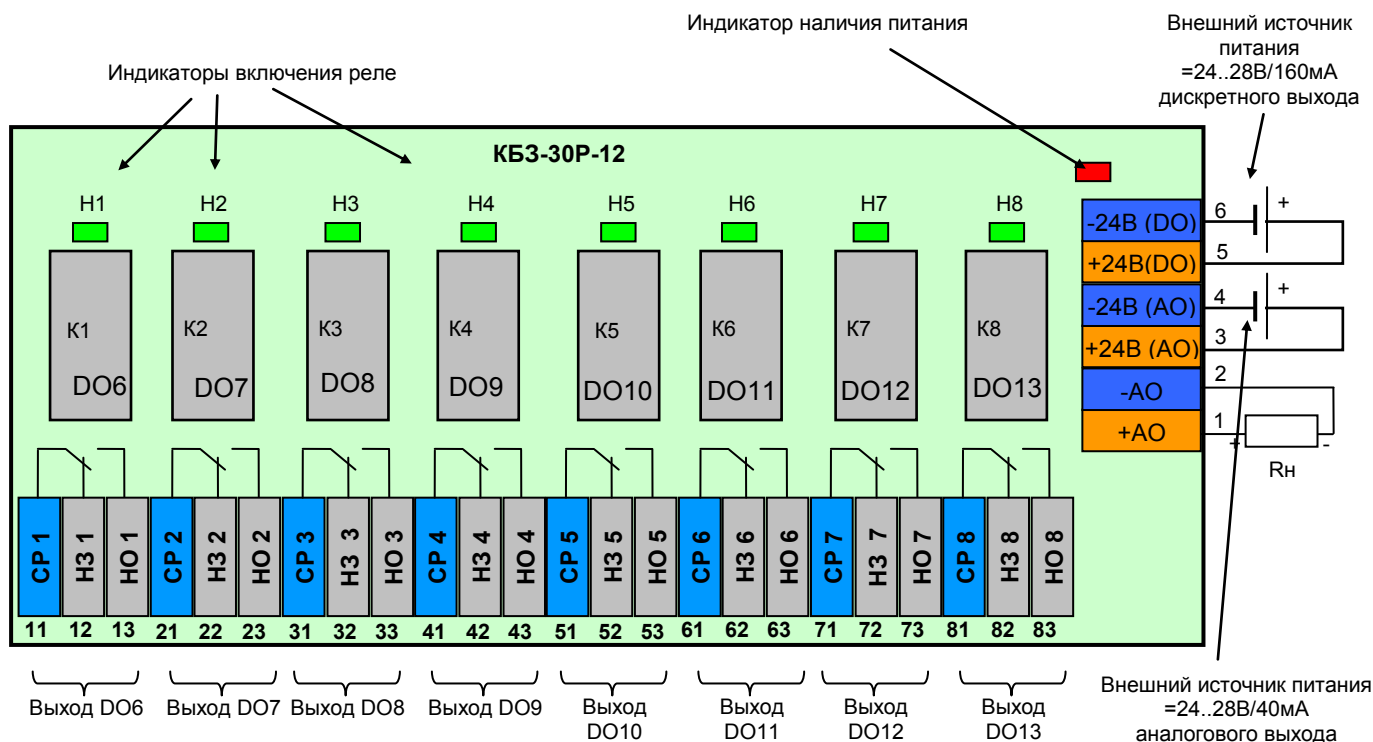
Рисунок 10.4.6.2 - Подключение сигналов модуля расширения МР-51-06 с помощью клеммно-блочного соединителя KB3-30P-12
