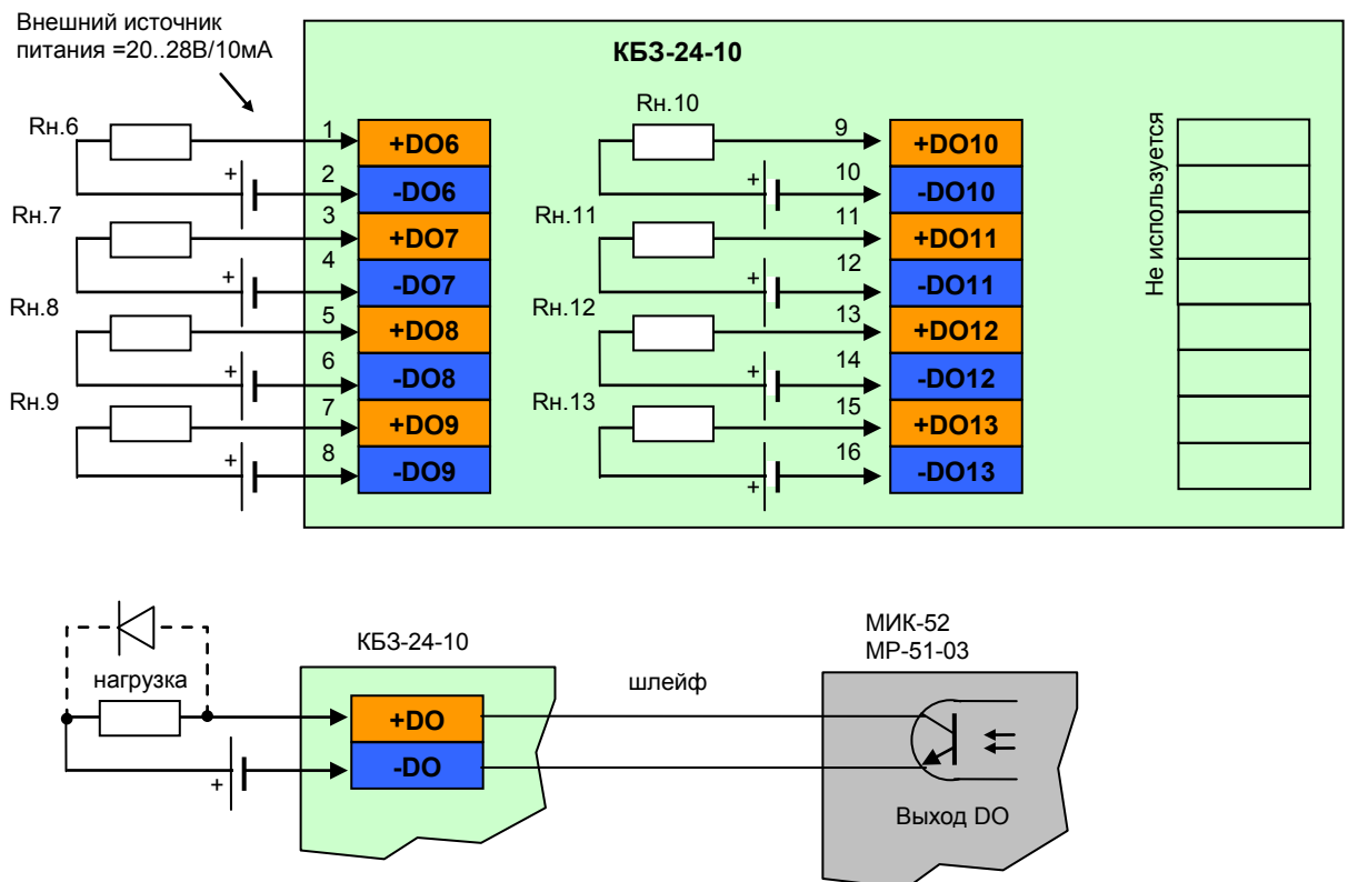
Рисунок 10.4.3.1 - Подключение сигналов модуля расширения МР-51-03 с помощью клеммно-блочного соединителя КБ3-24-10
