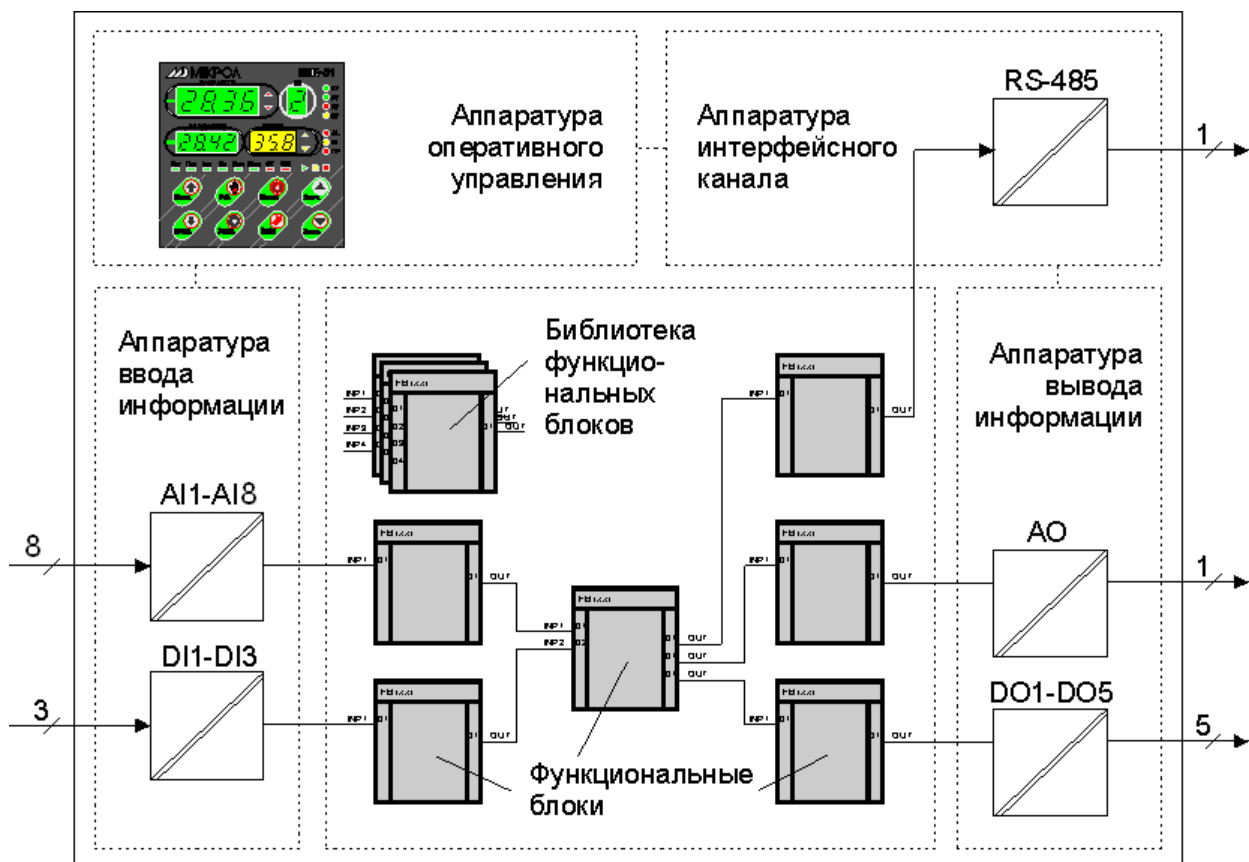
Рисунок 4.1 - Архитектура контроллера МИК-52
