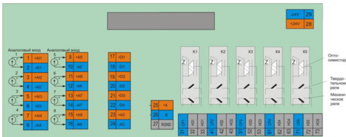
Рисунок 10.2 - Подключение аналоговых входов с помощью клеммно-блочного соединителя КБ3-34Р-01, КБ3-34К-01, КБ3-34С-01.
