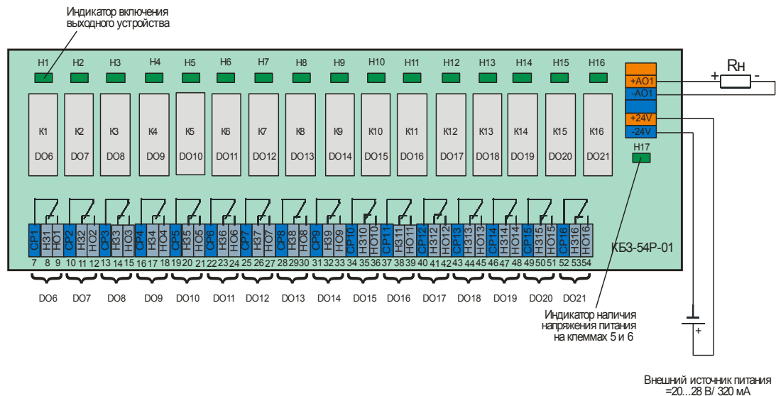
Рисунок 10.4.11.2 - Подключение сигналов модуля расширения МР-51-15 с помощью клеммно-блочного соединителя КБ3-54Р-01
