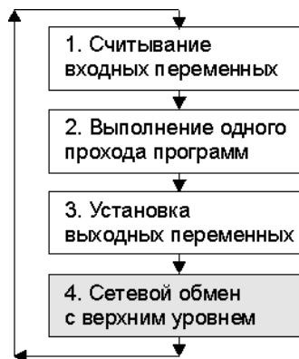
Рисунок 4.7 - Циклограмма работы контроллера
