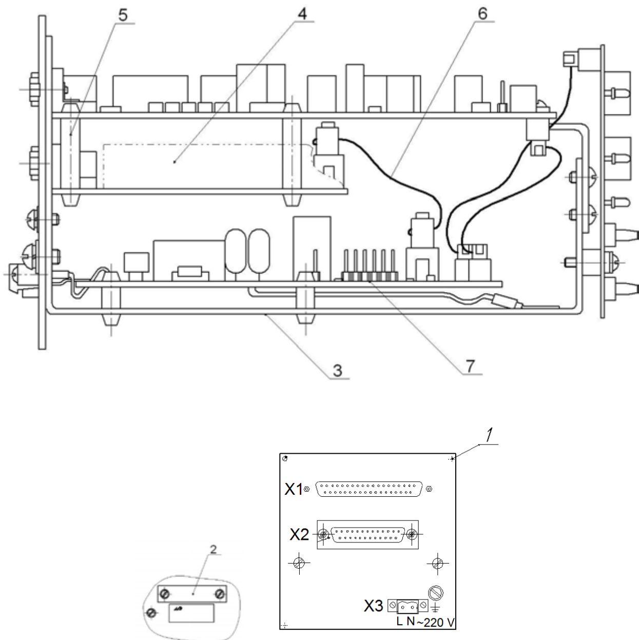
Рисунок 9.2 – Установка модуля расширения МР-51
