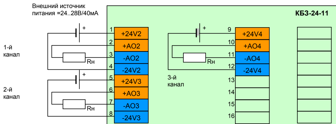
Рисунок 10.4.7 - Подключение сигналов модуля расширения МР-51-07 с помощью клеммно-блочного соединителя KB3-24-11
