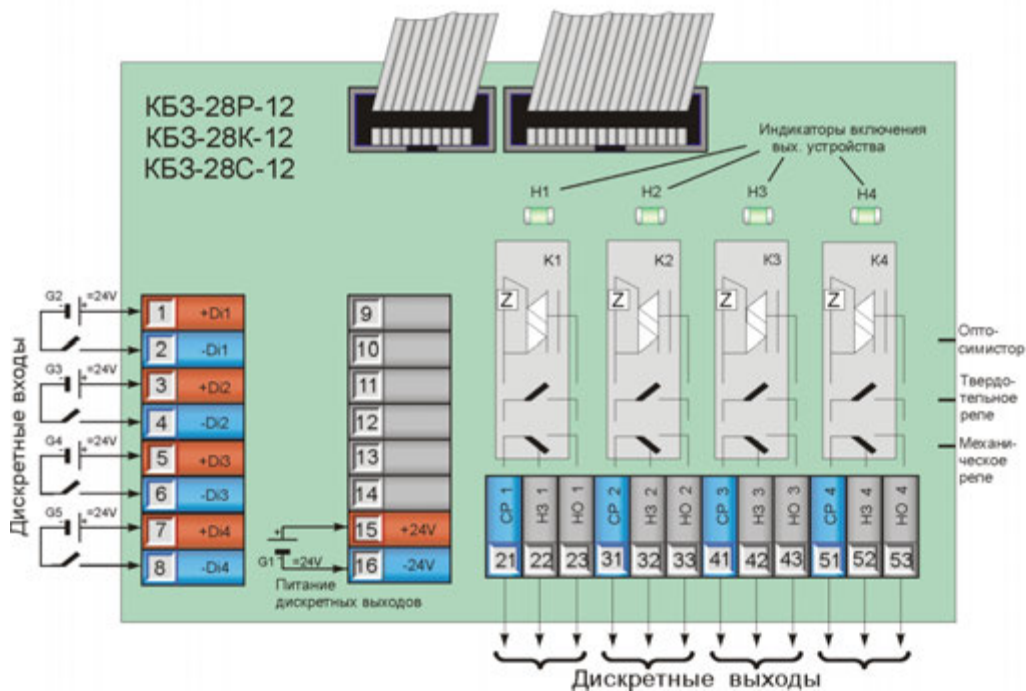
Рисунок 10.4.2.2 - Подключение сигналов модуля расширения МР-51-02 с помощью клеммно-блочного соединителя КБ3-28Р-12, КБ3-28С-12, КБ3-28К-12
