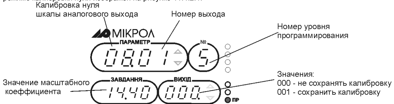
Рис 11.4.2.1 Внешний вид индикаторов при калибровке нуля аналогового выхода
