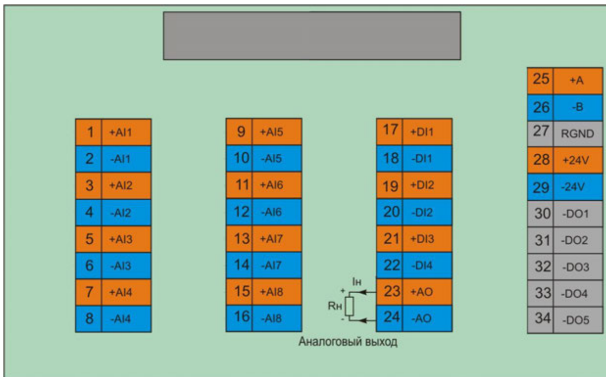
Рисунок 10.6 - Подключение аналоговых выходов с помощью клеммно-блочного соединителя КБЗ-34-01
