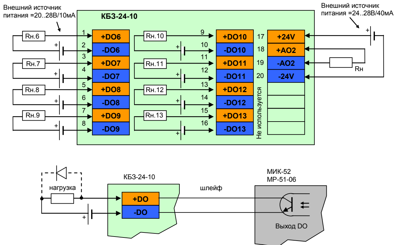
Рисунок 10.4.6 - Подключение сигналов модуля расширения МР-51-06 с помощью клеммно-блочного соединителя KB3-24-10
