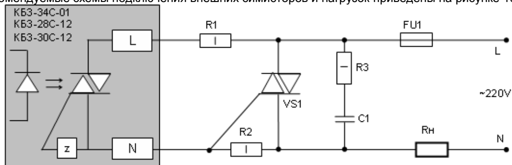
Рисунок 10.10 – Схема подключения внешнего симистора
