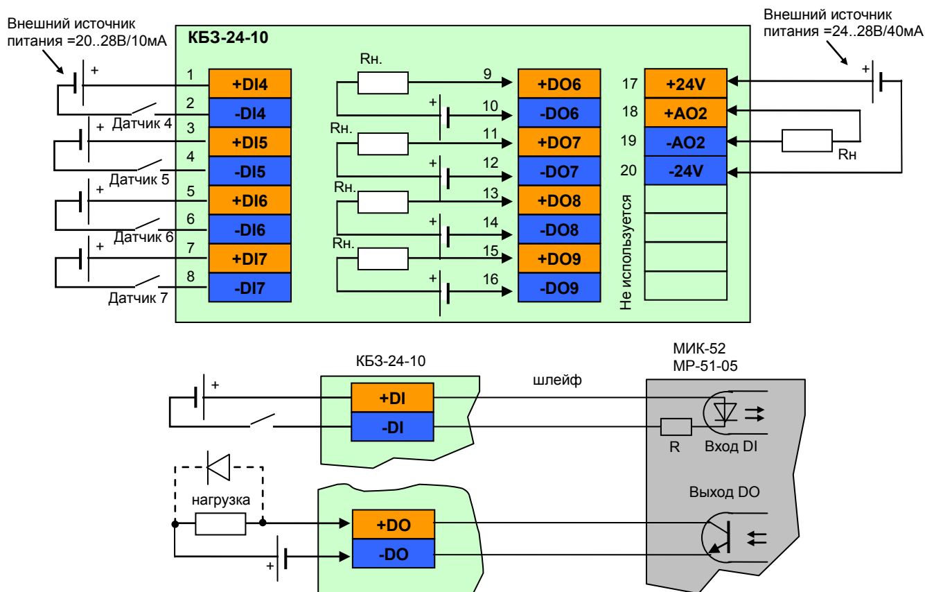
Рисунок 10.4.5.1 - Подключение сигналов модуля расширения МР-51-05 с помощью клеммно-блочного соединителя КБ3-24-10
