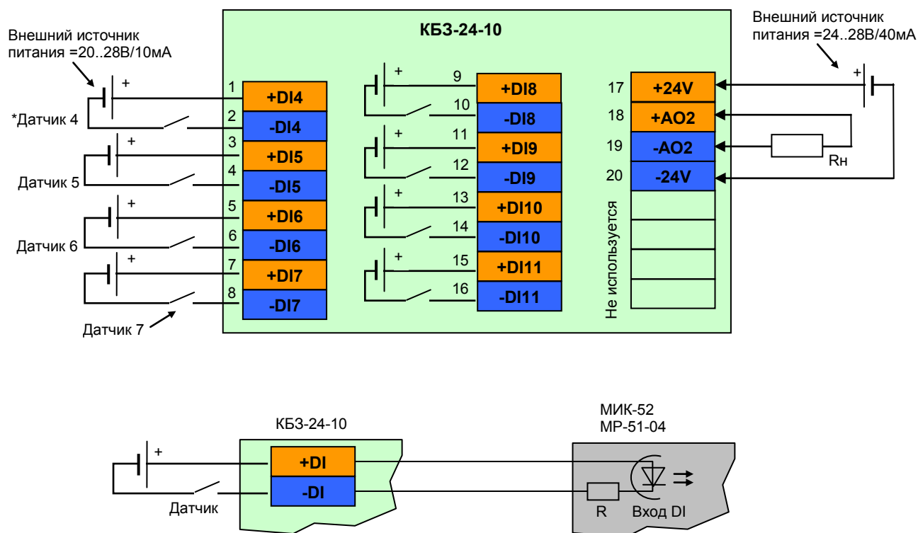
Рисунок 10.4.4.1 - Подключение сигналов модуля расширения MP-51-04 с помощью клеммно-блочного соединителя KB3-24-10
