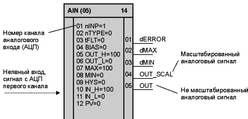
Рисунок 4.3 - Функциональный блок аналогового ввода с неявными входами
