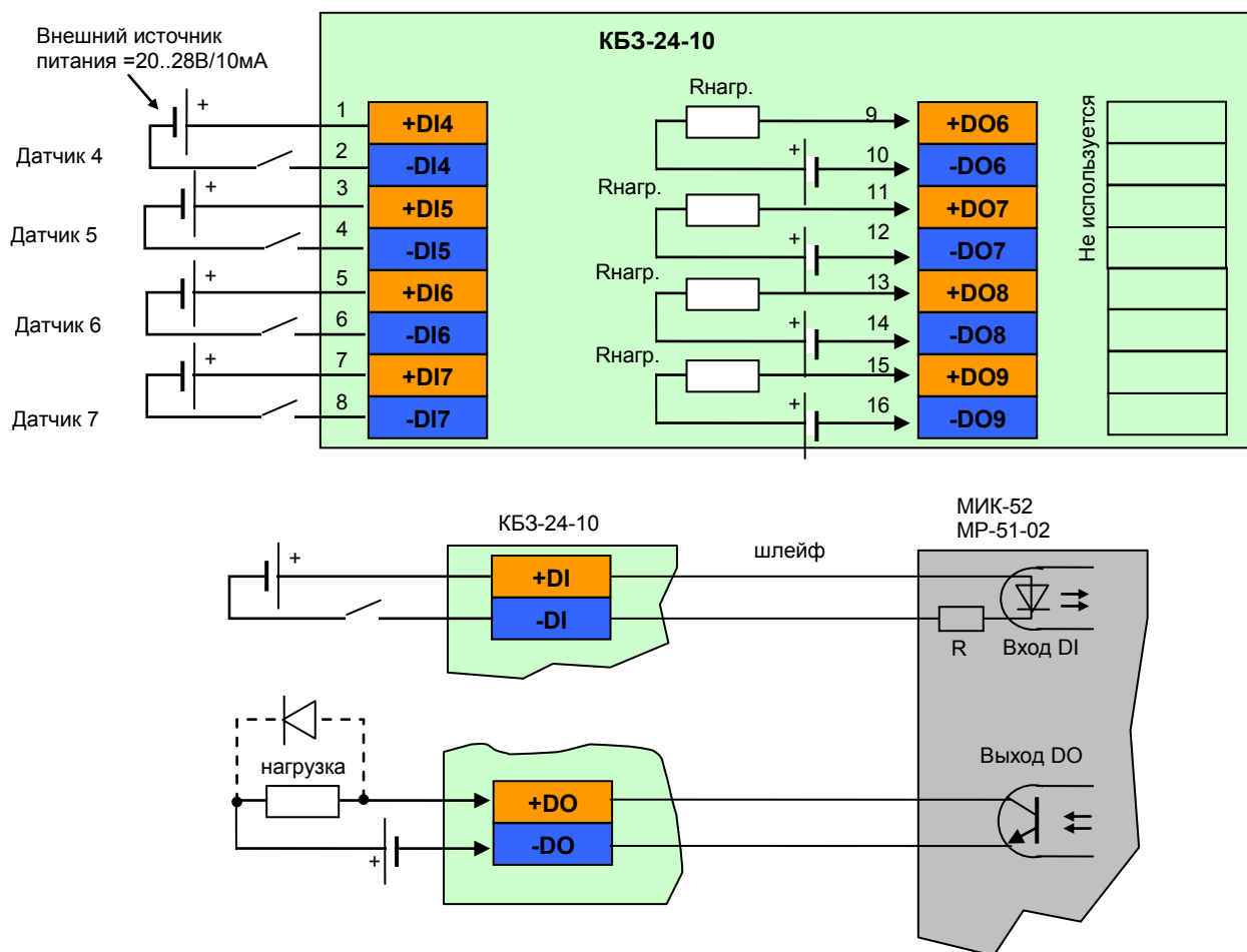
Рисунок 10.4.2.1 - Подключение сигналов модуля расширения МР-51-02 с помощью клеммно-блочного соединителя KB3-24-10
