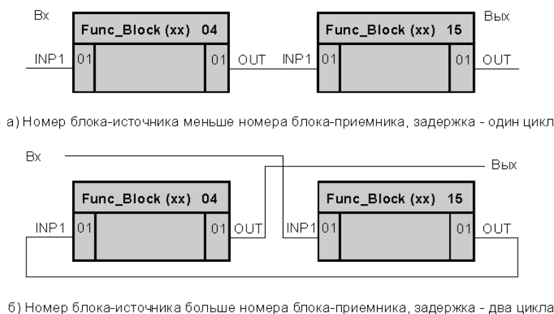
Рисунок 4.8 - Задержка обслуживания
