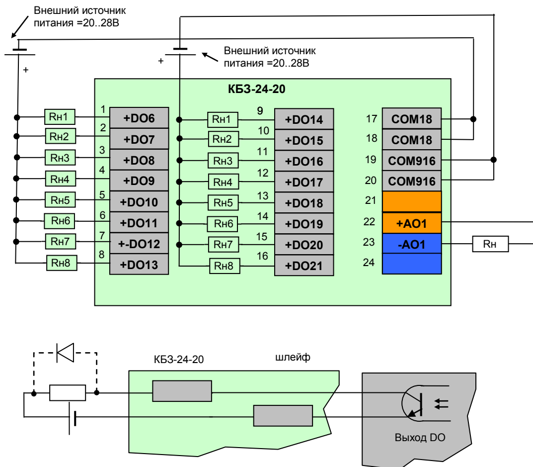
Рисунок 10.4.10.1 - Подключение сигналов модуля расширения МР-51-15 с помощью клеммно-блочного соединителя KB3-24-20
