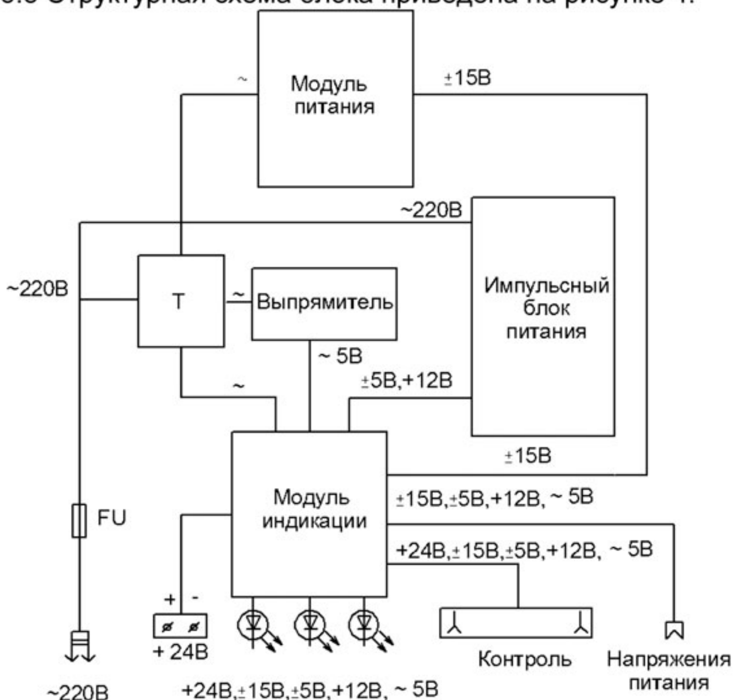
Рисунок 4 – Блок питания стабилизирующий БПС-7. Схема структурная.
