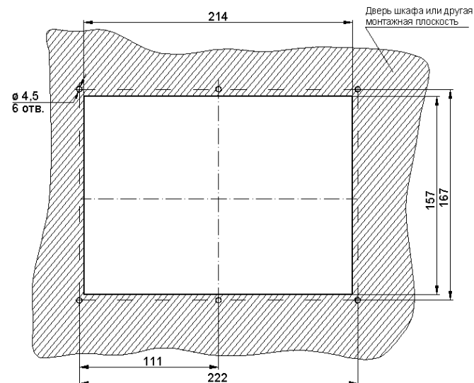
Рисунок 1 – Размеры окна для установки панели
