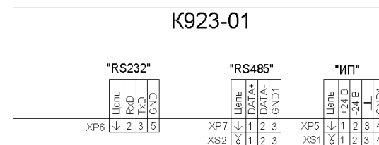
Рисунок 2 – Схема подключения панели
