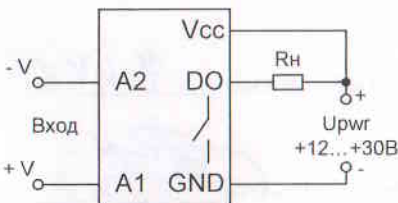
д) питание модуля и нагрузки от источника питания 12...30В
