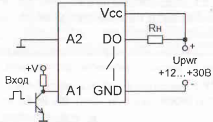
г) выходной транзистор открыт, управление NPN транзистором
