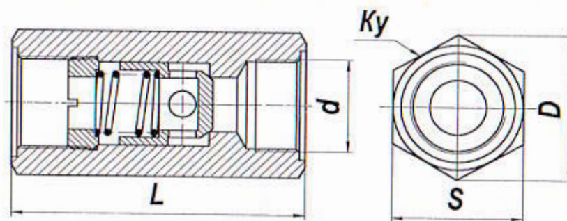
Рисунок 2-основные габаритные и присоединительные размеры клапана обратного
