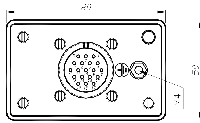
Рисунок 6 - Габаритные размеры ДРТ-Ж-...-M24
