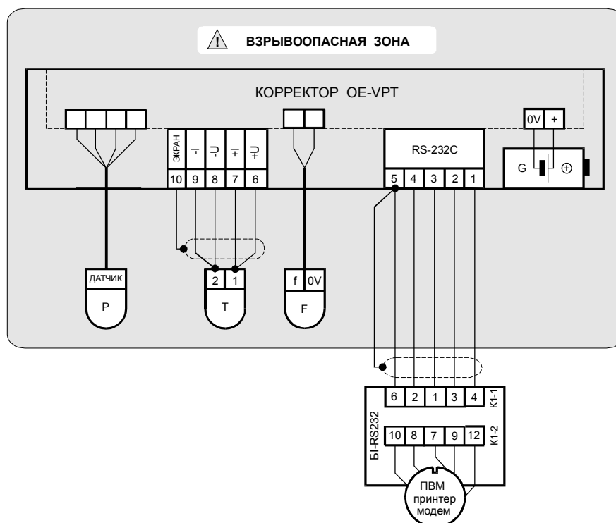
Рисунок 9.2 – Монтаж внешних цепей корректора и блока интерфейса BI-RS232 при установке корректора во взрывоопасной зоне
