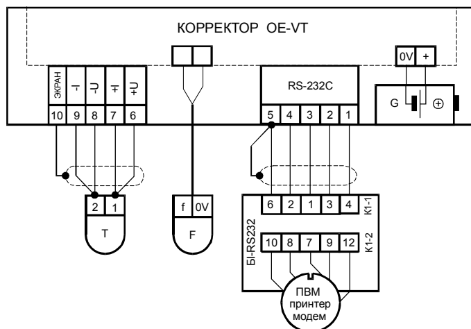
Рисунок 9.1 – Монтаж внешних цепей корректора и блока интерфейса BI-RS232
