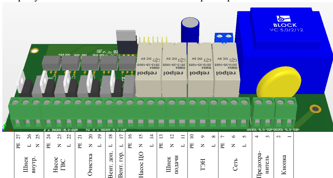
Рисунок 6 – Подключение нагрузок к силовой плате.
