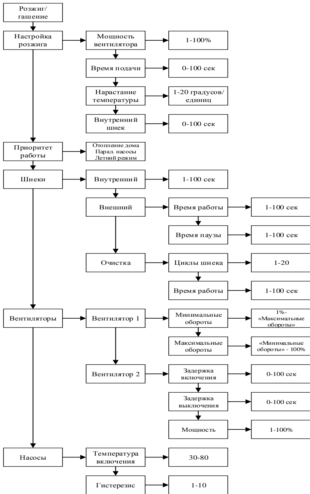
Рисунок 7 – Структура меню
